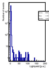
RAYRAWW2 ch08 (cable 031)
