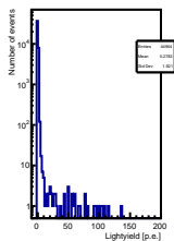
RAYRAWW2 ch16 (cable 037)
