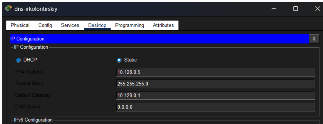
Рис. 2: Настройка IP DNS-сервера
