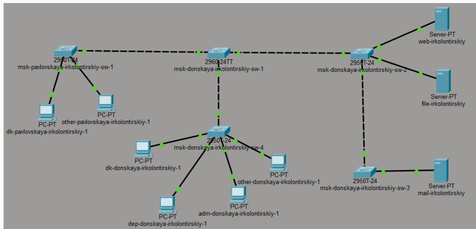
Рис. 1: Схема L1
