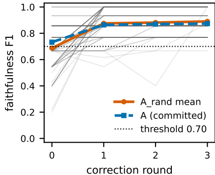
F1 per round
