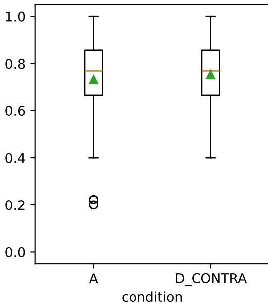
Faithfulness F1
