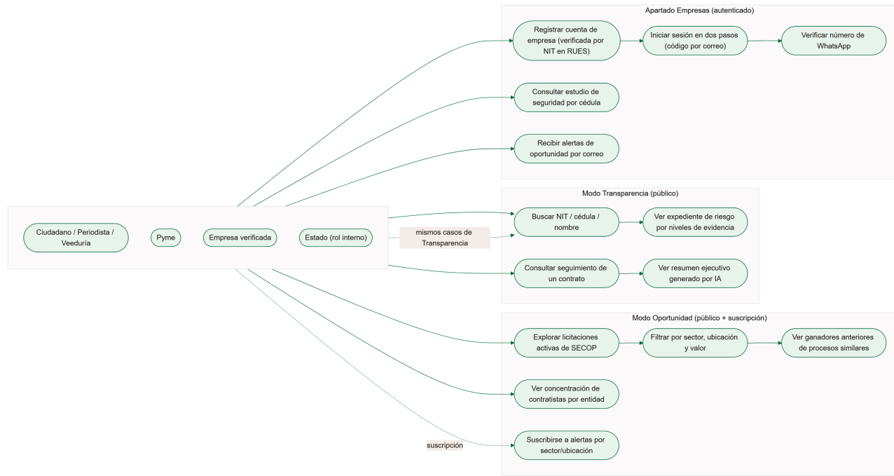
Figura 1 — Casos de uso por actor.
