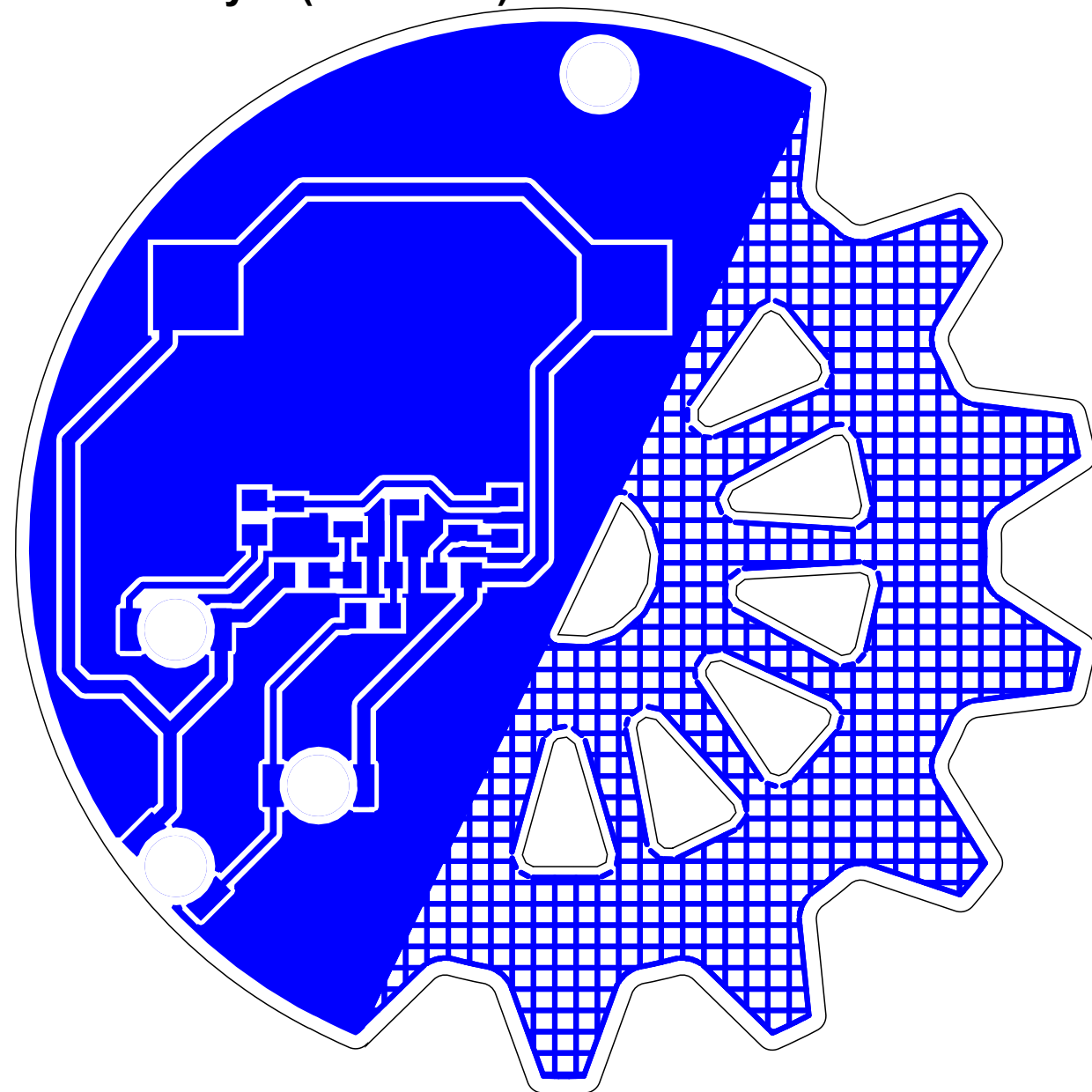
Bottom Layer (Scale 4:1)
