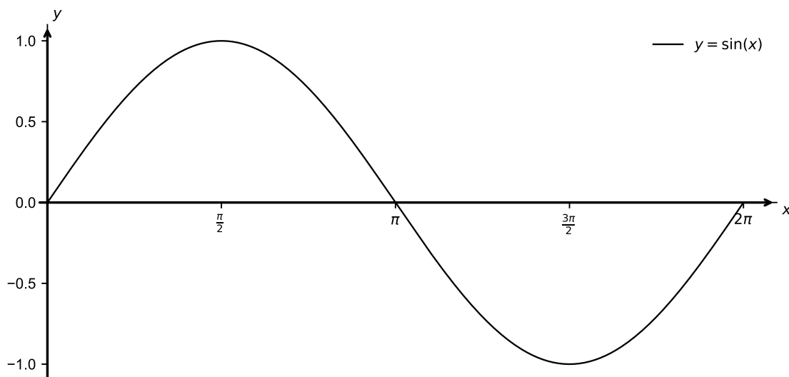
Rys. 3.1. Wykres funkcji sinus. Kod programu w Pythonie wykres znajduje siǎ w Dodatku A.
