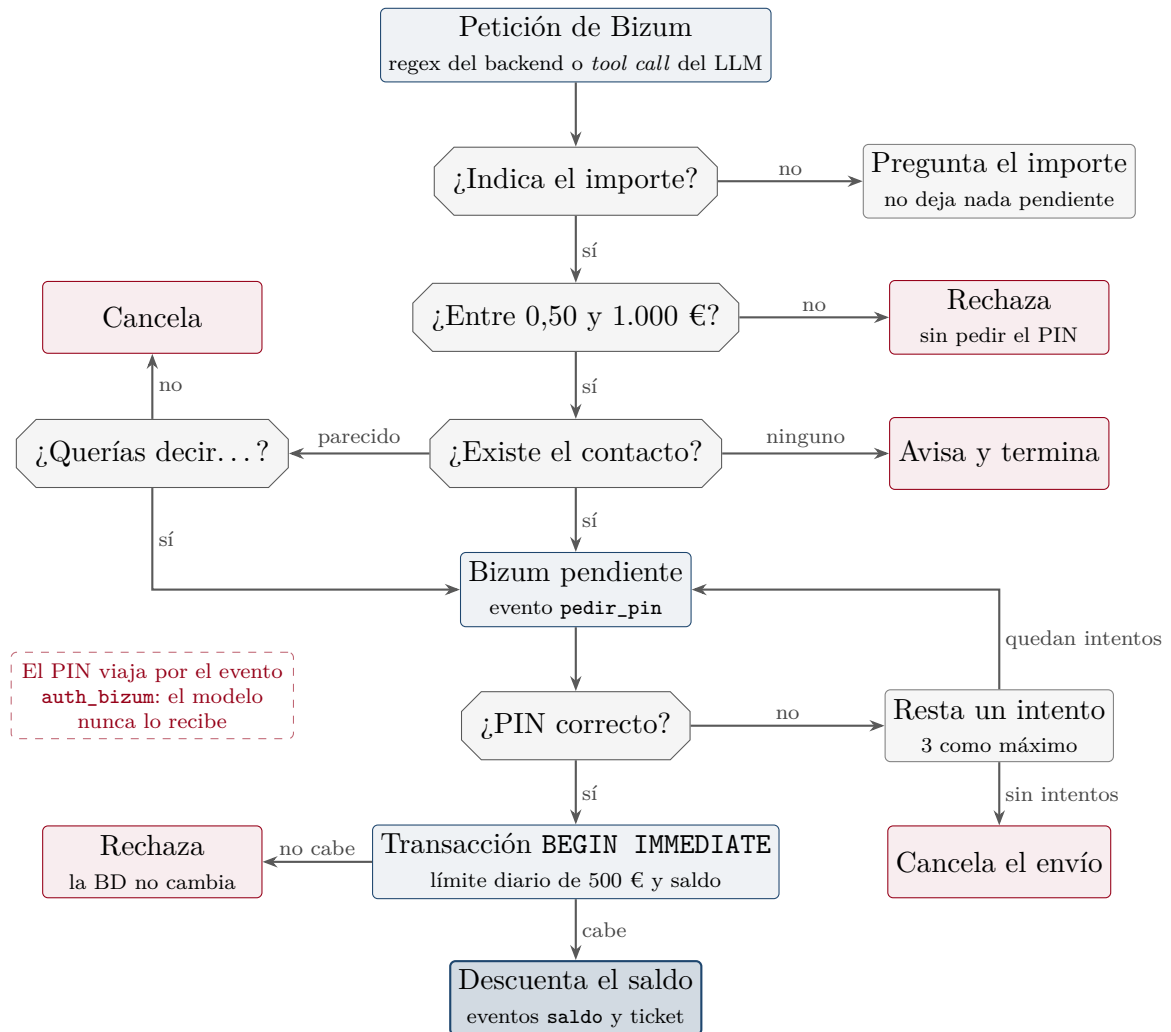
Figura 3: Flujo de un envío de Bizum. Todas las comprobaciones se hacen en el backend y en este orden: el importe se valida antes de pedir el PIN, y el límite diario y el saldo se comprueban dentro de la misma transacción que los descuenta.
