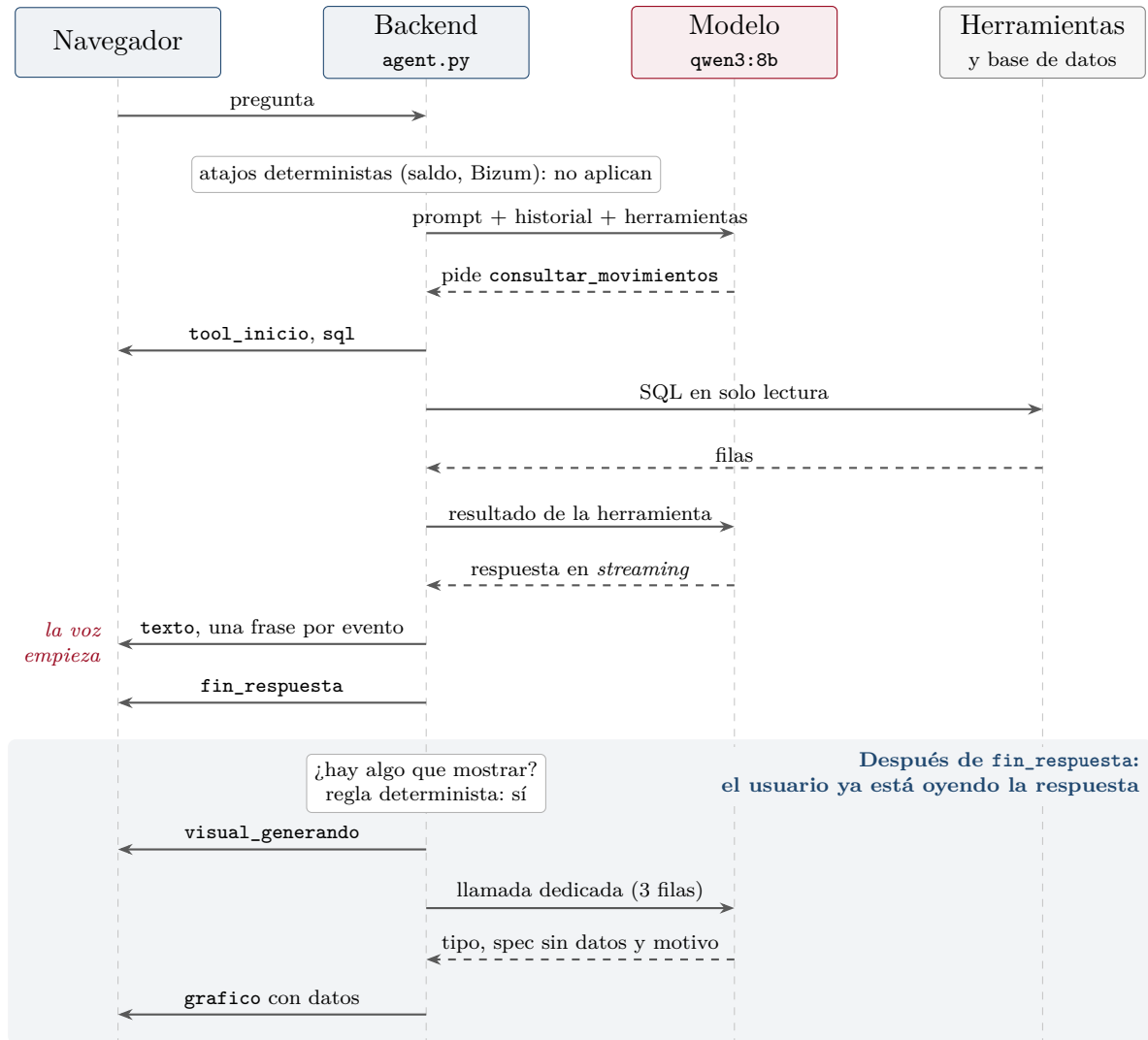
Figura 2: Secuencia de un turno con consulta al histórico y gráfico. La voz empieza con la primera frase del texto. El motor visual solo se ejecuta cuando la respuesta ya está completa, de modo que la segunda llamada al modelo no retrasa lo que el usuario oye.
