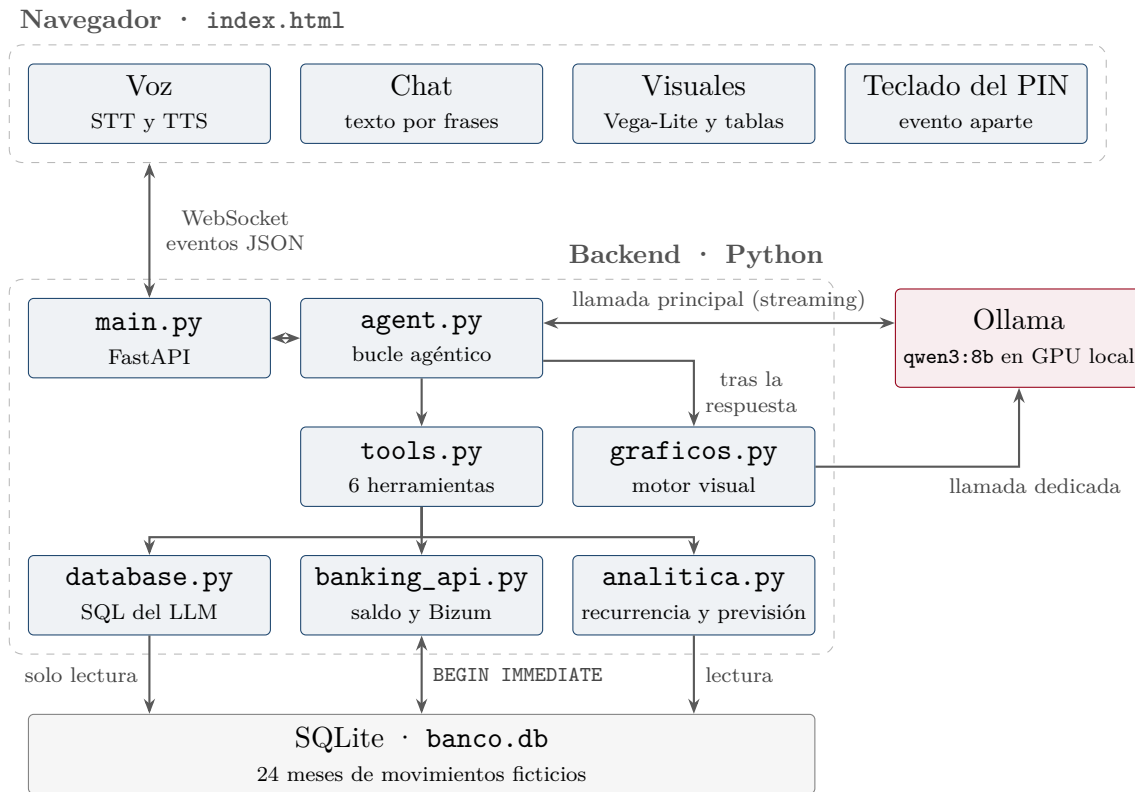
Figura 1: Arquitectura del sistema. El modelo se ejecuta en local y el backend es el único que accede a la base de datos: el SQL generado por el LLM entra por una conexión de solo lectura, y las escrituras solo se hacen desde las APIs bancarias, dentro de una transacción.
