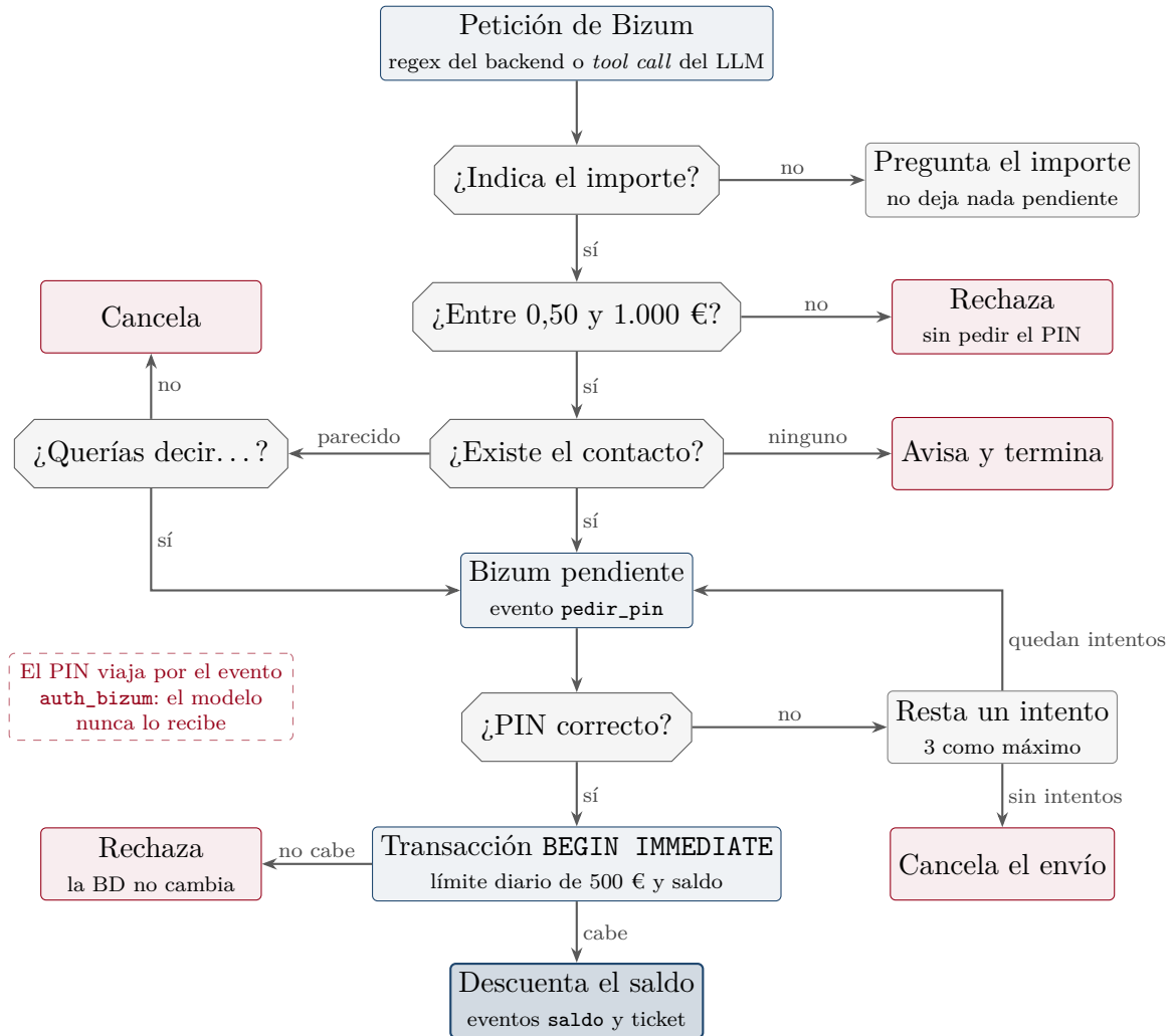
Figura 4: Flujo de un envío de Bizum. Todas las comprobaciones se hacen en el backend y en este orden: el importe se valida antes de pedir el PIN, y el límite diario y el saldo se comprueban dentro de la misma transacción que los descuenta.
