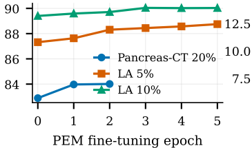
Dice (%) \uparrow
