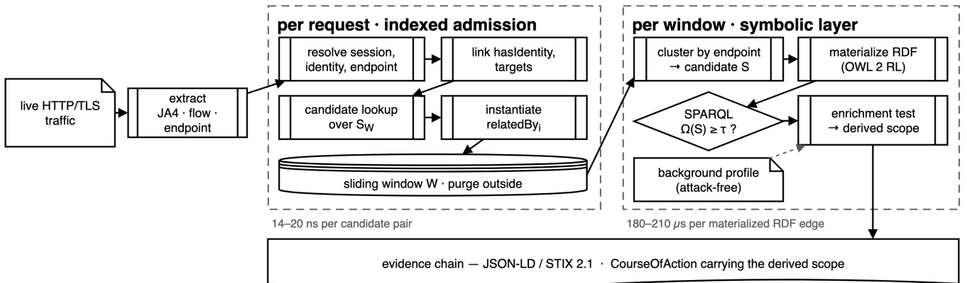
Fig. 2. O pipeline de execução, e a divisão que torna seu custo suportável. As duas camadas operam em taxas diferentes: a admissão é por requisição, sobre índices invertidos, enquanto a materialização RDF e a agregação de \Omega acontecem uma vez por janela, quatro ordens de grandeza adiante por unidade de trabalho. O teste de enriquecimento lê um perfil de fundo construído fora de episódios de ataque, de modo que nenhum rótulo entra no caminho de decisão em momento algum.
