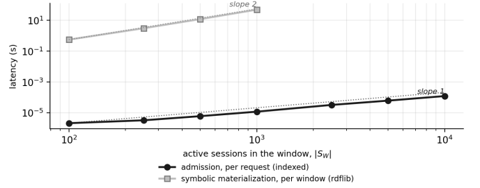
Fig. 5. Custo das duas camadas em função da ocupação da janela. A admissão por requisição é linear em |S_W| e permanece na faixa de microssegundos; a materialização simbólica por janela é linear no número de arestas RDF, que por sua vez é quadrático em |S_W| . Retas de referência ancoradas no primeiro ponto de cada série.
