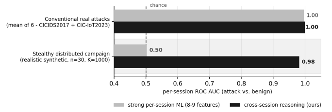
Fig. 4. Onde o raciocínio entre sessões é necessário . Em ataques reais convencionais um classificador por sessão forte já satura; só no regime furtivo distribuído a detecção por sessão colapsa para o acaso enquanto o raciocínio entre sessões se sustenta.
