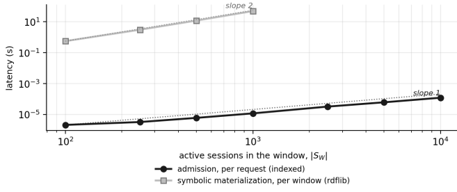
Fig. 5. Custo das duas camadas em função da ocupação da janela. A admissão por requisição é linear em |S_W| e permanece na faixa de microssegundos; a materialização simbólica por janela é linear no número de arestas RDF, que por sua vez é quadrático em |S_W| . Retas de referência ancoradas no primeiro ponto de cada série.
