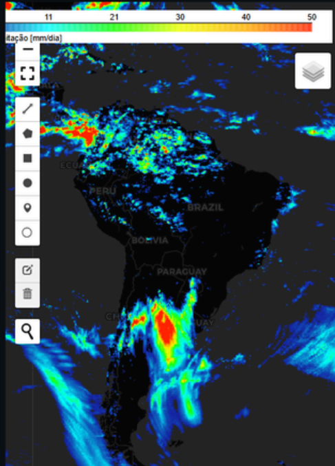
IMERG
