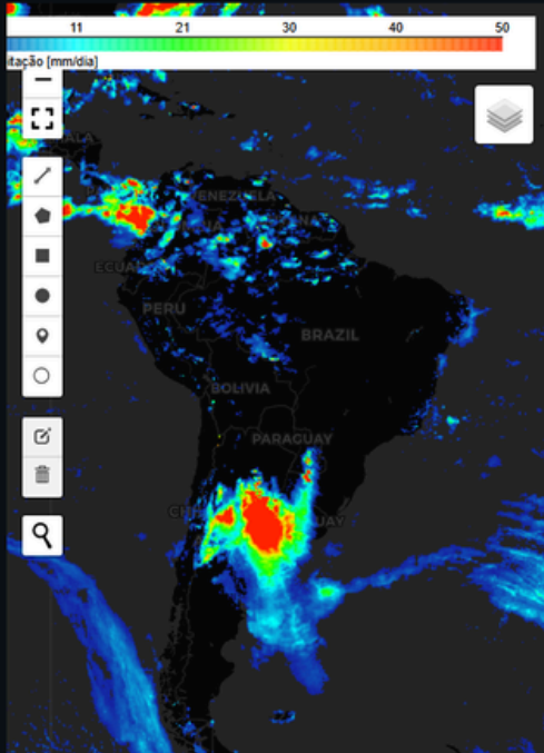
GSMaP
