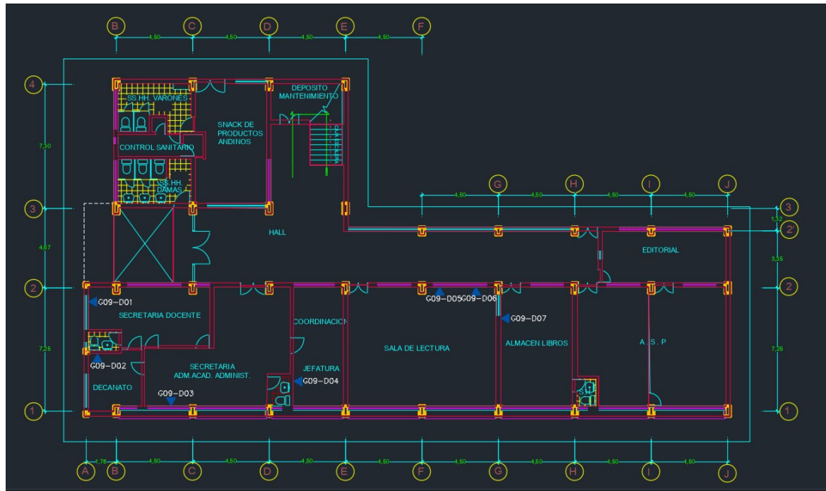
Figura 2.3: Plano del primer nivel con puntos de red G09-D01 a G09-D07 y rutas de canalización. Esc. 1:100.
