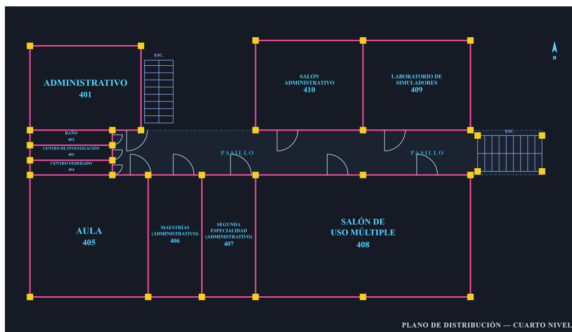
Figura 6 Plano del cuarto nivel con puntos de red G09-D14 a G09-D29 y ubicación del Gabinete G09 (MDF). Esc. 1:100.
