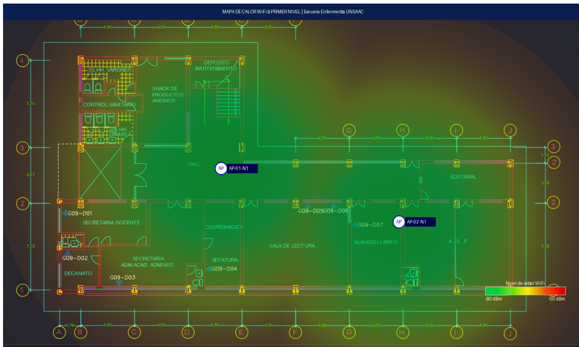
Figura 11 Mapa de calor WiFi — Primer nivel. AP-01-N1 en hall central y AP-02-N1 en sala de lectura. Escala cromática: verde ( \geq -50 dBm, excelente) a rojo (zona muerta, < -85 dBm).
