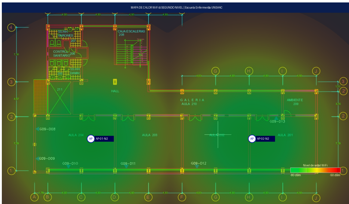
Figura 12 Mapa de calor WiFi — Segundo nivel. AP-01-N2 cubre aulas 203/204 y AP-02-N2 cubre aulas 201/202. Se aprecia el solapamiento de celdas (15–20 %) necesario para roaming continuo.
