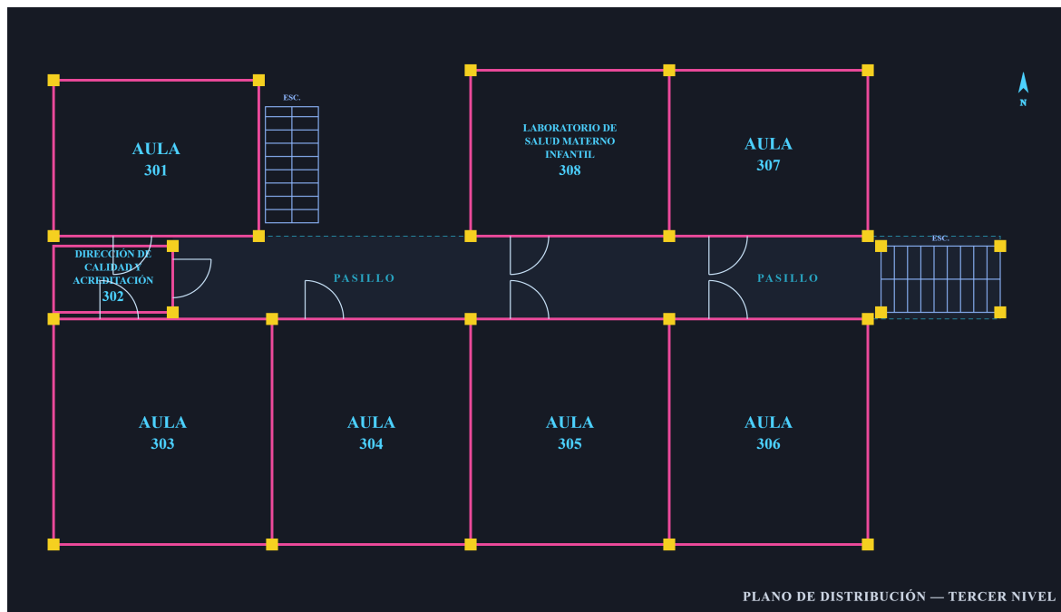
Figura 5 Plano del tercer nivel con puntos de red G09-D14 a G09-D22 y rutas de canalización. Esc. 1:100.
