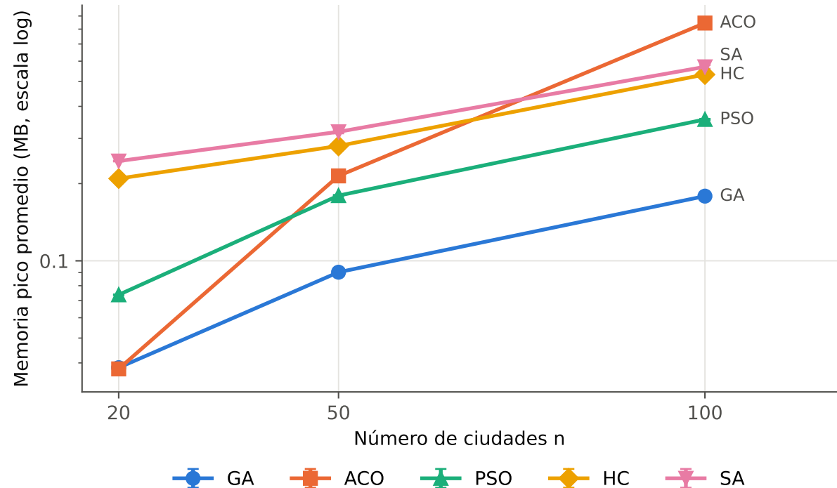
Memoria máxima (tracemalloc) frente al número de ciudades
