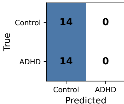
Always-Control
