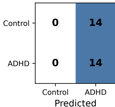
Always-ADHD
