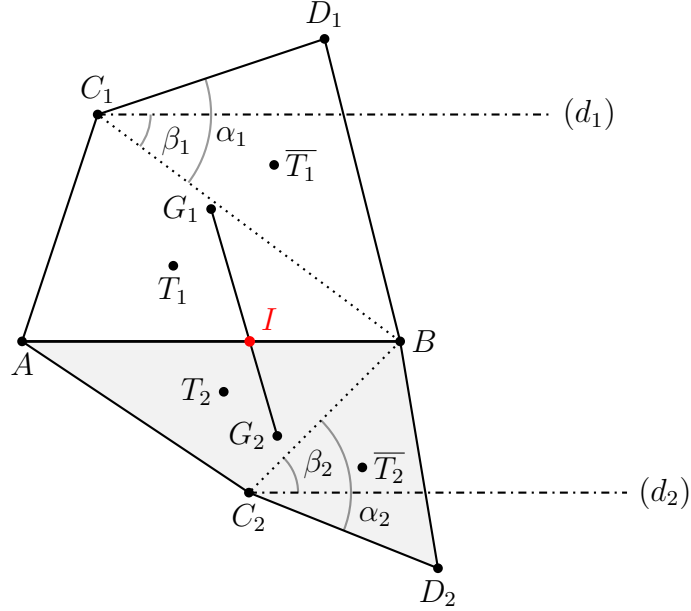
FIGURE 9 – Deux quadrangle ABD_1C_1 et ABD_2C_2 de centre de gravité G_1 et G_2 respectivement. Les points T_k et \overline{T}_k sont les centres de gravités de ABC_k et BC_kD_k , et \alpha_k, \beta_k \in ]0, \pi[ .
