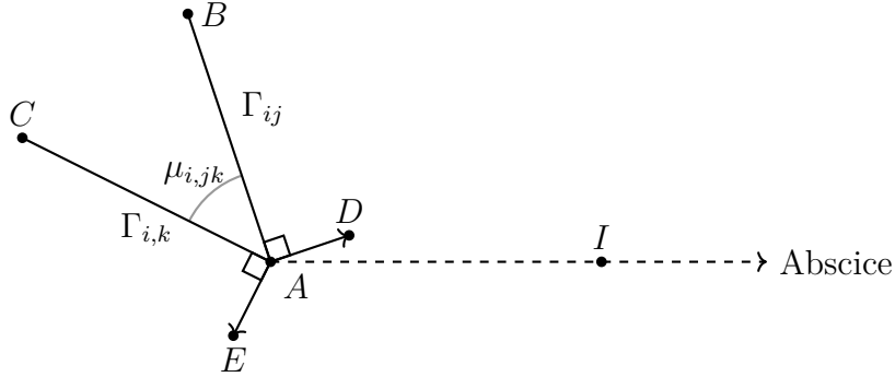
FIGURE 8 – Cellule C_i représenté avec les interfaces \Gamma_{ij} = [AB] et \Gamma_{i,k} = [AC] . Le vecteur \vec{AD} (resp. \vec{AE} ) est le vecteur n_{ij} (resp. n_{i,k} ). De plus I est un point placé sur l'abscisse avec une abscisse positive, où A est le centre du repère.
