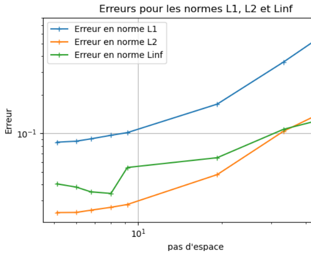
(b) Maillages quadrangulaires de déformation \varphi = 0.5 .
