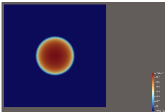
Figure 2: Fonction plateau.
