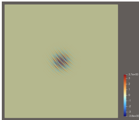
Figure 2: Fonction anisotrope.
