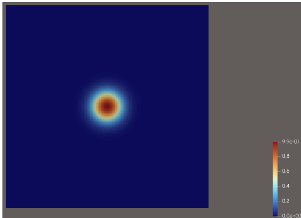
Figure 2: Gaussienne.
