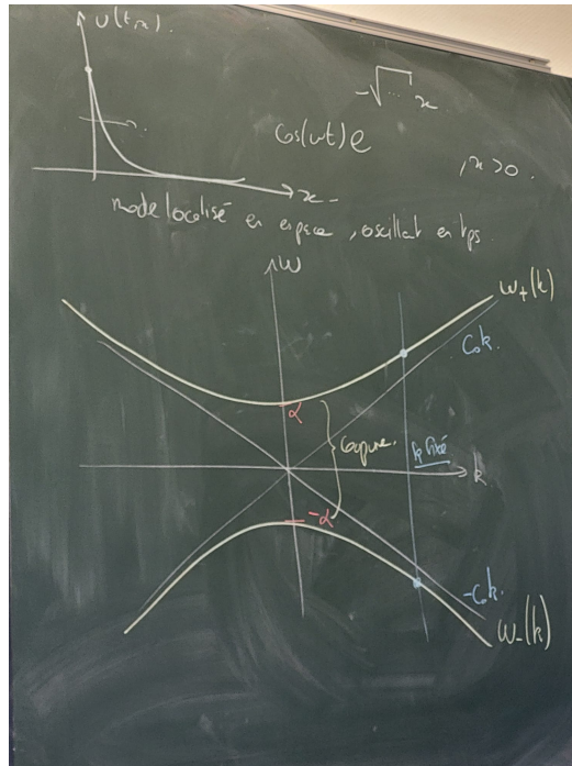
FIGURE 9 – Visualisation des solutions de l'exemple 6.
