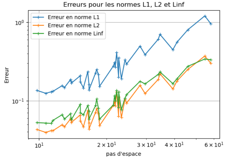
(b) Graphique en échelle logarithmique pour u^1
