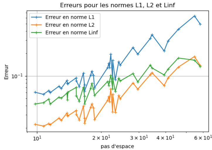
(c) Graphique en échelle logarithmique pour u^2
