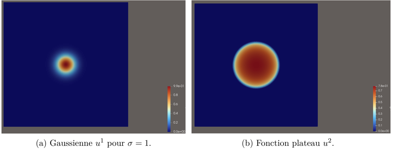
FIGURE 11 – Fonctions tests sur [0, 10] \times [0, 10] .
