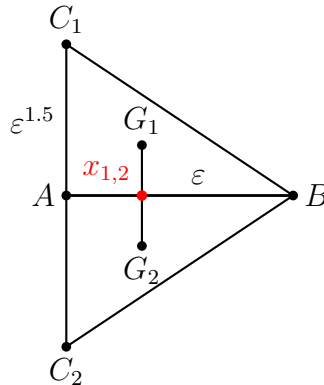
FIGURE 4 – Maillage \mathcal{T} constitués de deux triangle rectangles de taille \varepsilon \times \varepsilon^{1.5} . Avec, respectivement, G_1 et G_2 le centre de gravité de ABC_1 et ABC_2 .
