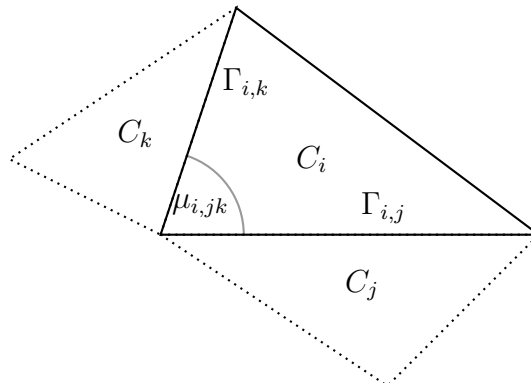
FIGURE 7 – Illustration d'une cellule C_i , avec \mu_{i,jk} \in ]0, \pi[ l'angle formé par \Gamma_{i,j} et \Gamma_{i,k} .
