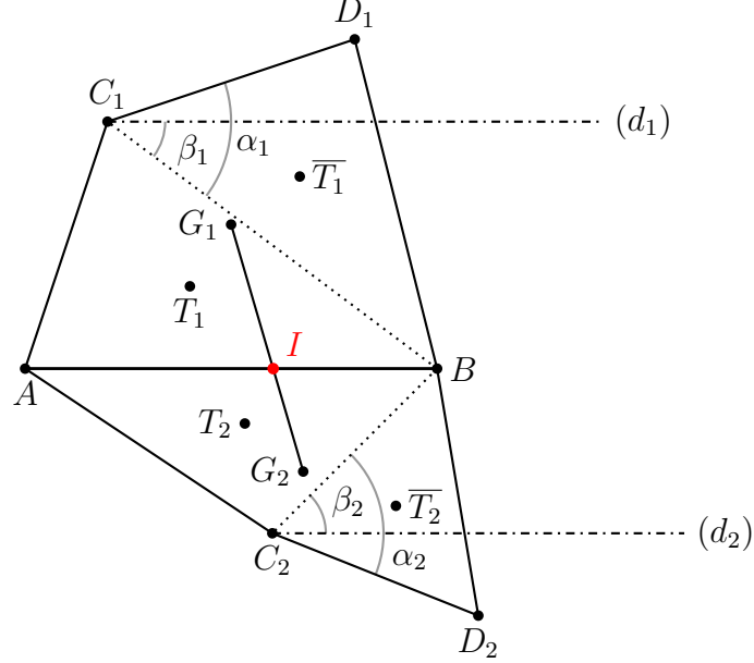
FIGURE 9 – Deux quadrangle ABD_1C_1 et ABD_2C_2 de centre de gravité G_1 et G_2 respectivement. Les points T_k et \overline{T}_k sont les centres de gravités de ABC_k et BC_kD_k , et \alpha_k, \beta_k \in ]0, \pi[ .
