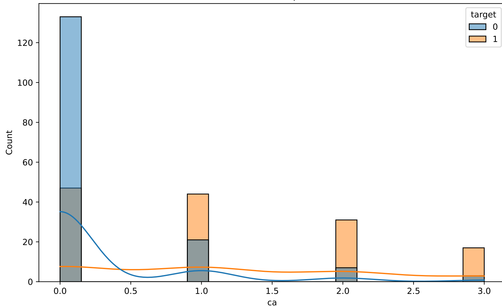
Distribution de ca par classe
