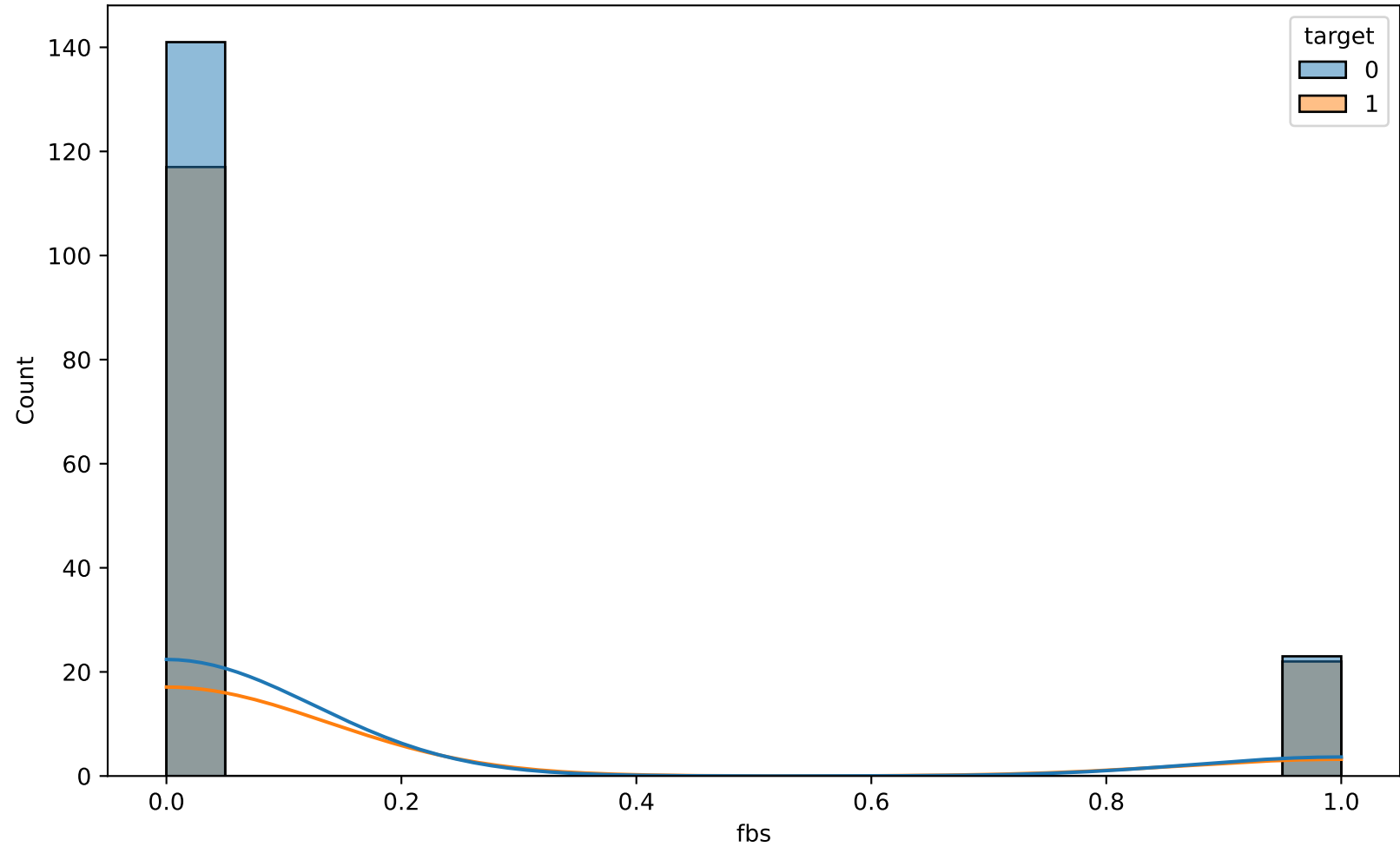
Distribution de fbs par classe
