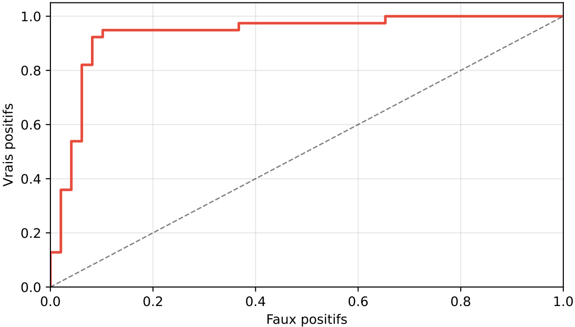
ROC (AUC = 0.934)
