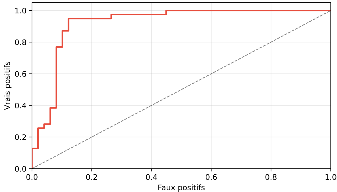
ROC (AUC = 0.920)
