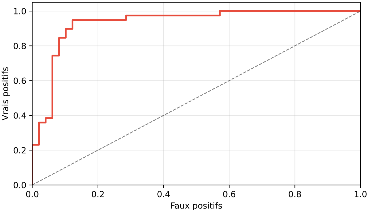
ROC (AUC = 0.932)
