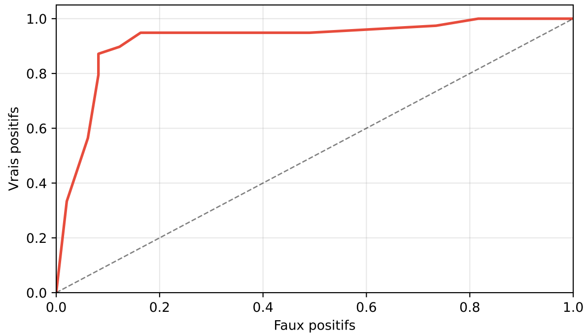
ROC (AUC = 0.919)
