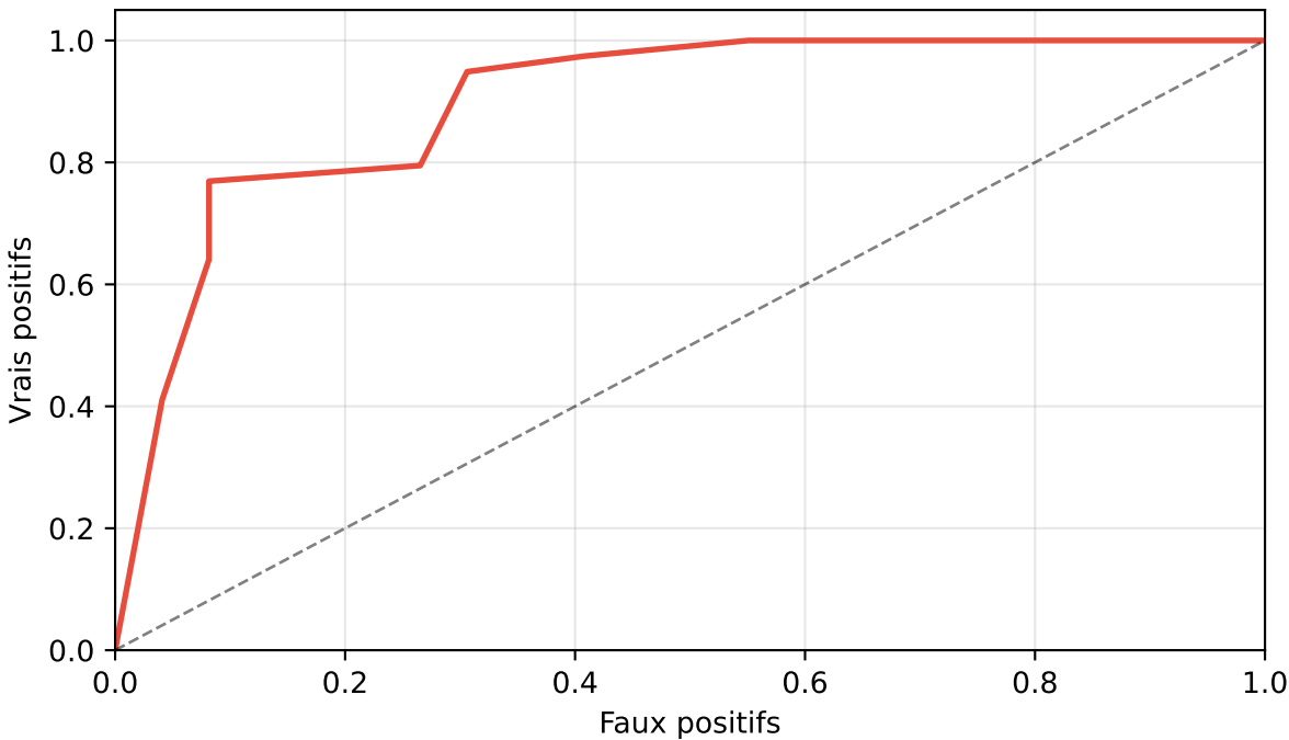
ROC (AUC = 0.897)
