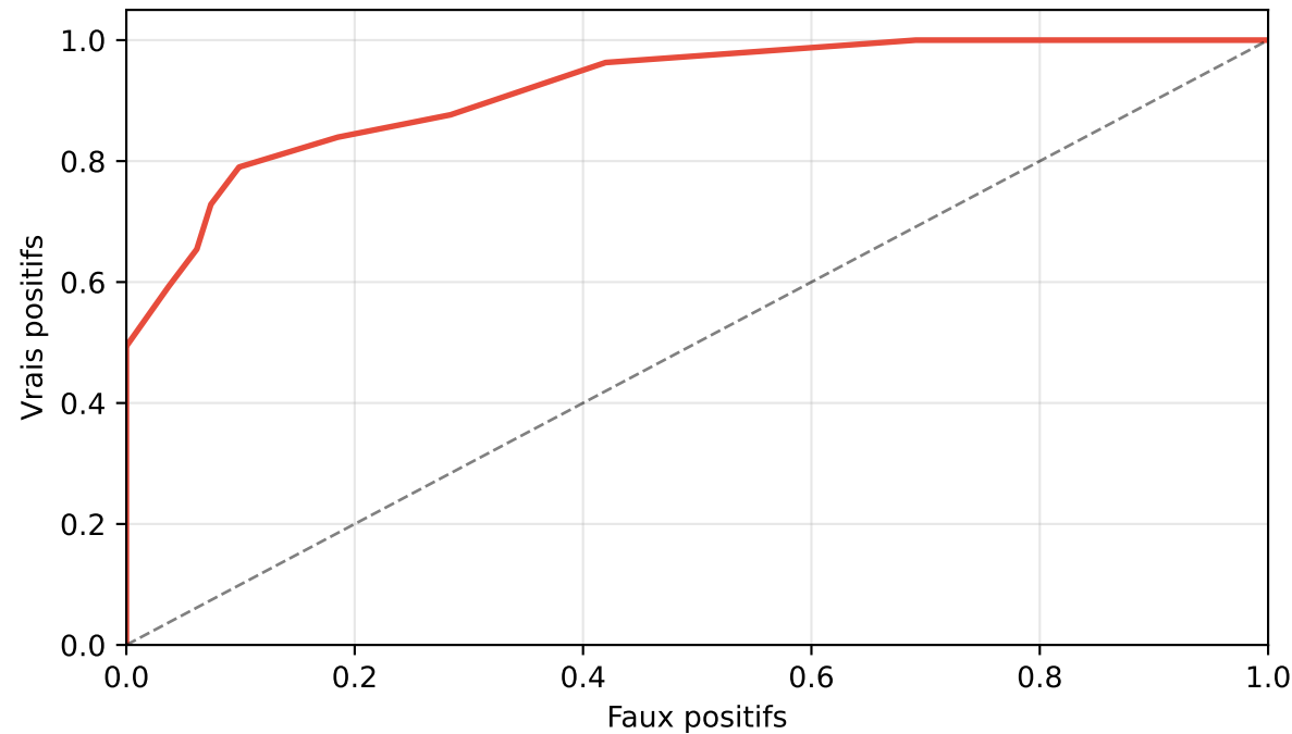
ROC (AUC = 0.918)
