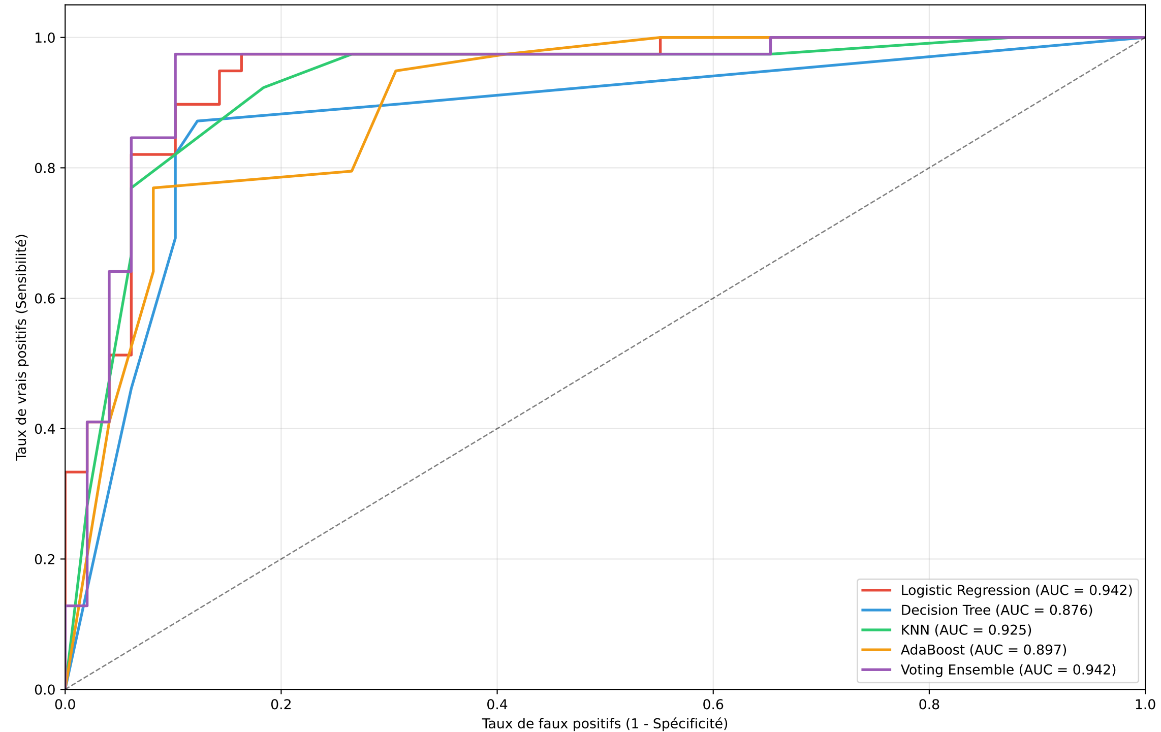
Courbes ROC des différents modèles
