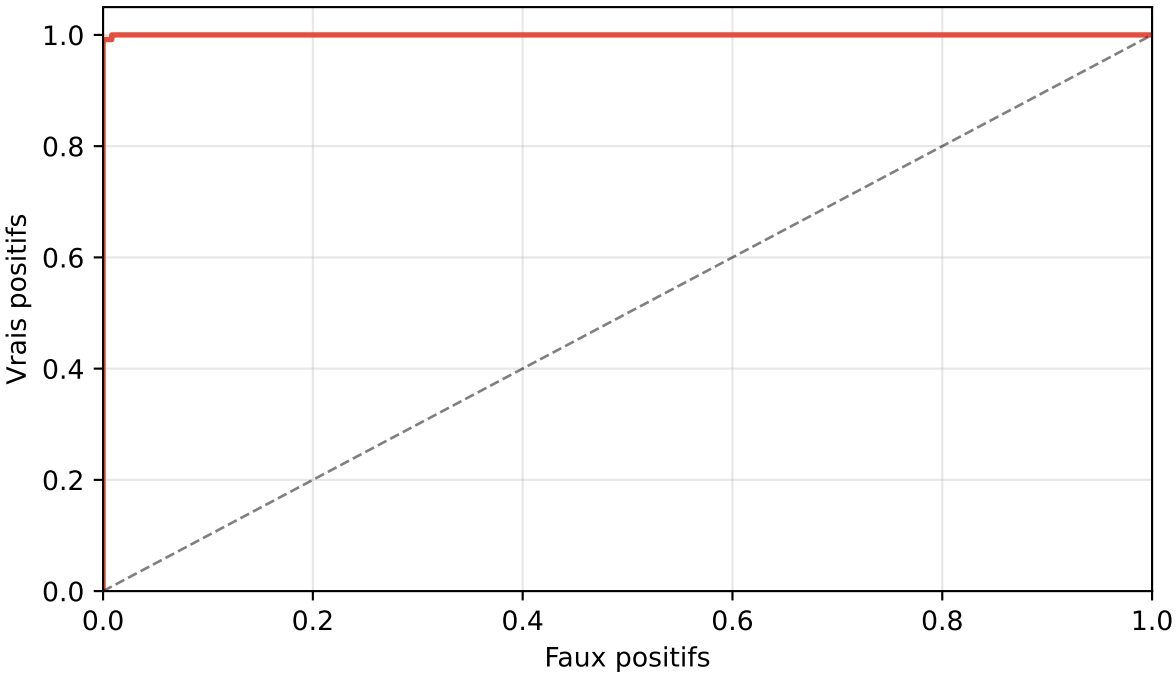
ROC (AUC = 1.000)
