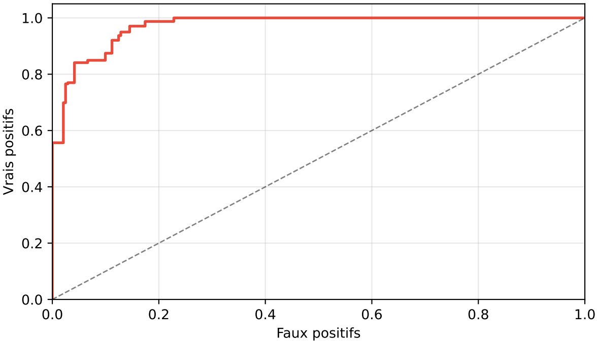
ROC (AUC = 0.972)
