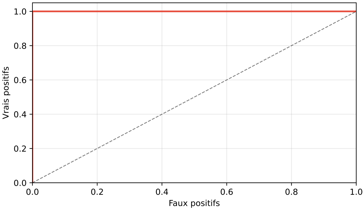
ROC (AUC = 1.000)
