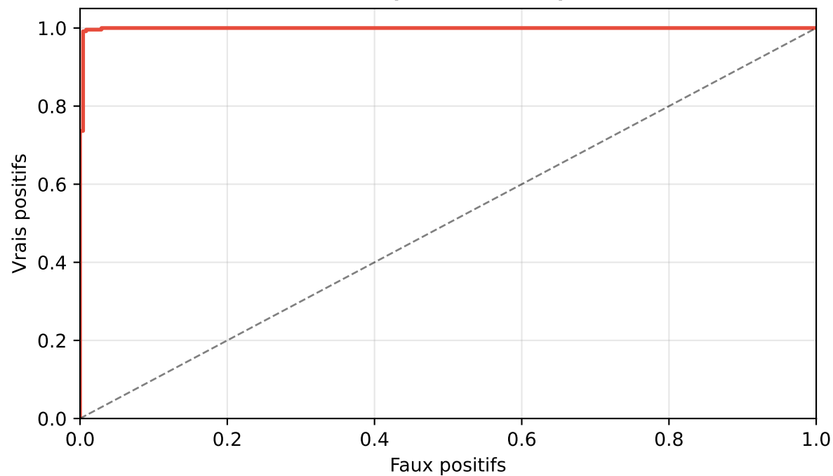
ROC (AUC = 0.999)
