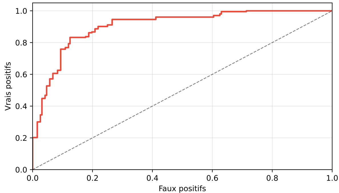
ROC (AUC = 0.906)
