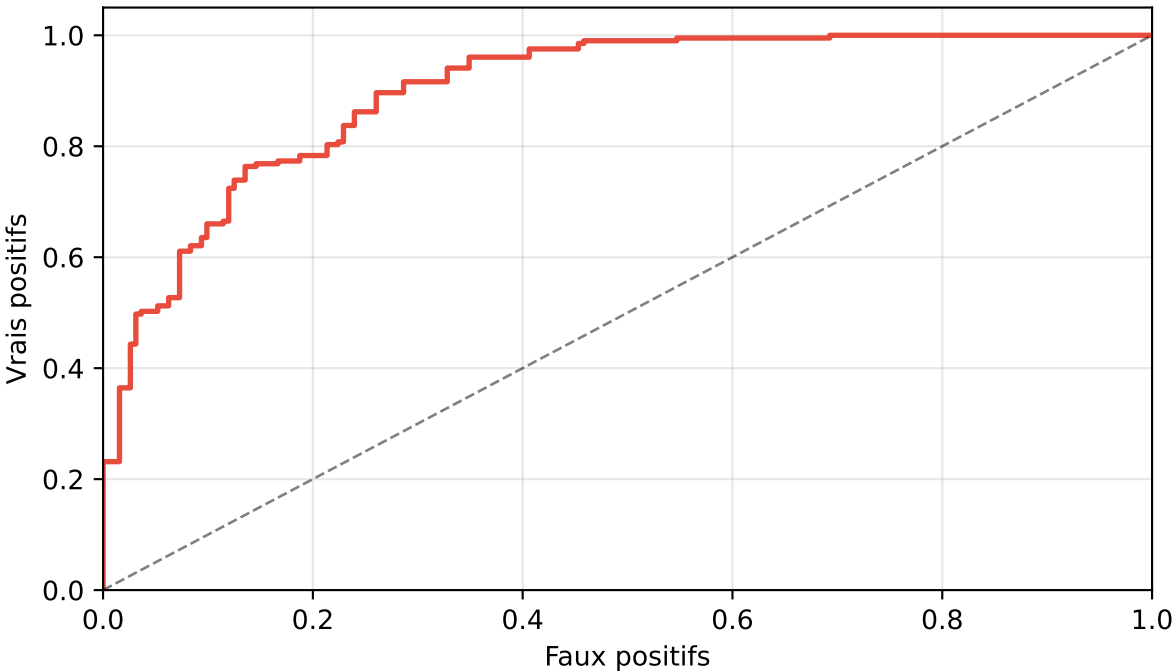
ROC (AUC = 0.899)
