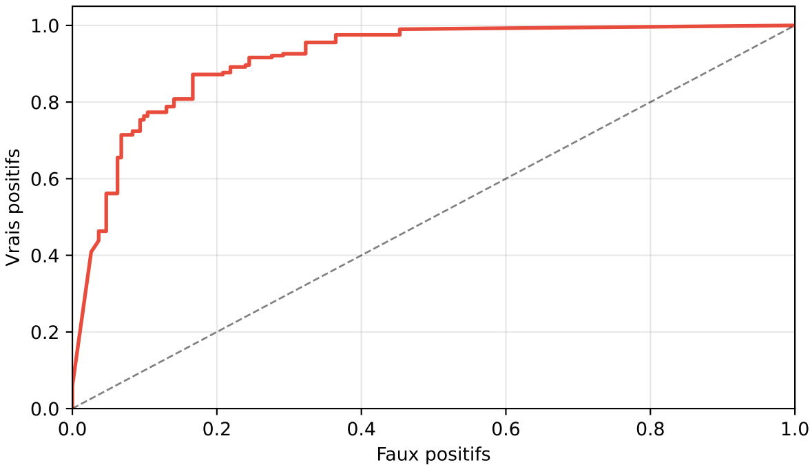
ROC (AUC = 0.915)
