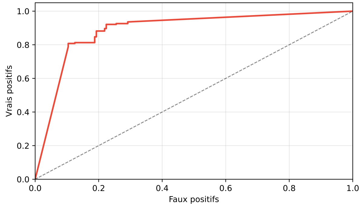
ROC (AUC = 0.889)
