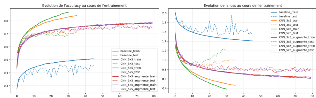
Figure 1 — Évolution de l'accuracy (gauche) et de la loss (droite) au cours de l'entraînement
