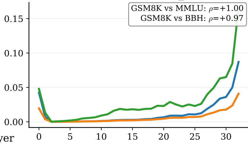
Mistral - Whitespace_10%
