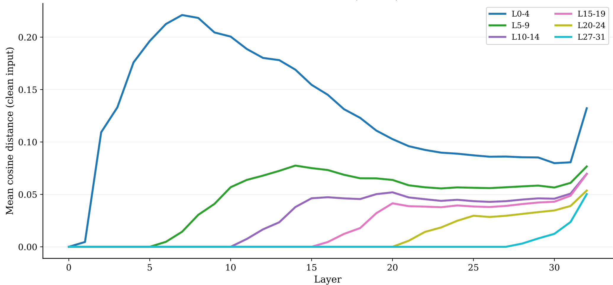
Mistral / GSM8K (n=200)
