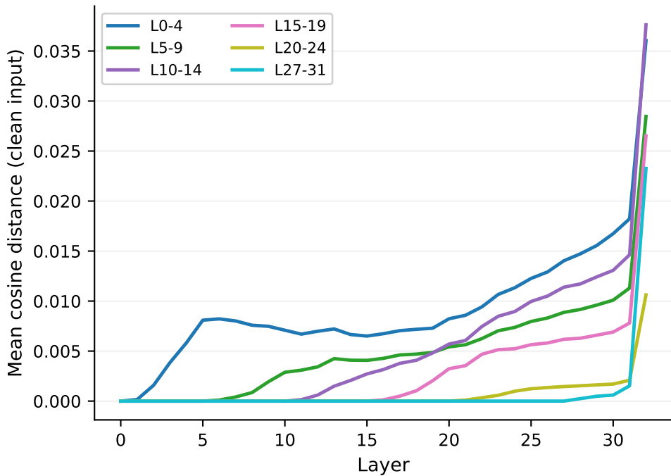
Phi-3.5-mini / GSM8K (n=200)
