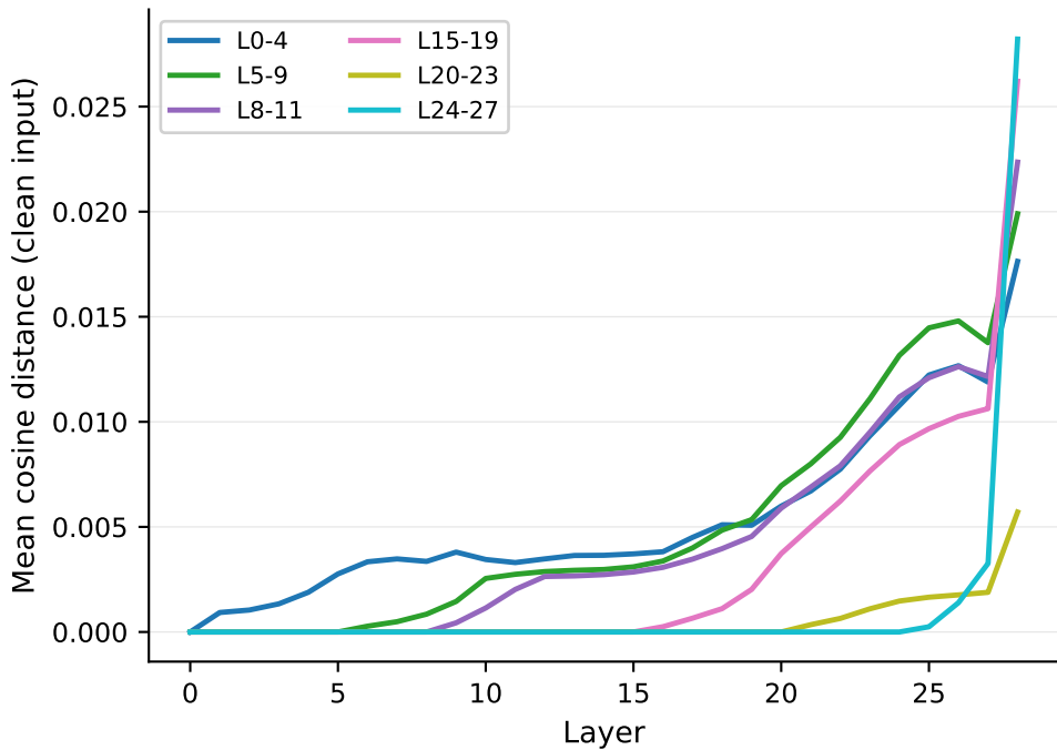
Qwen2.5-7B / GSM8K (n=200)
