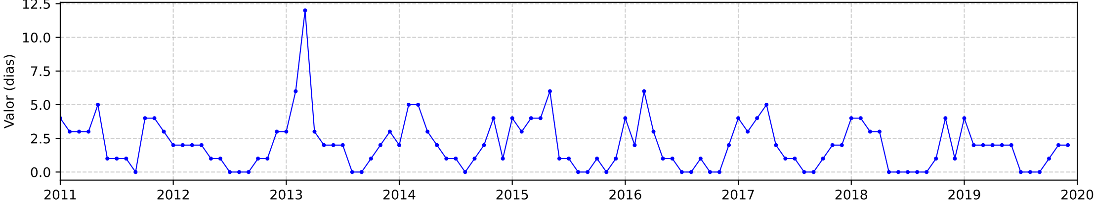
Estação: Barbalha, Década: 2011-2019, Índice: CWD
