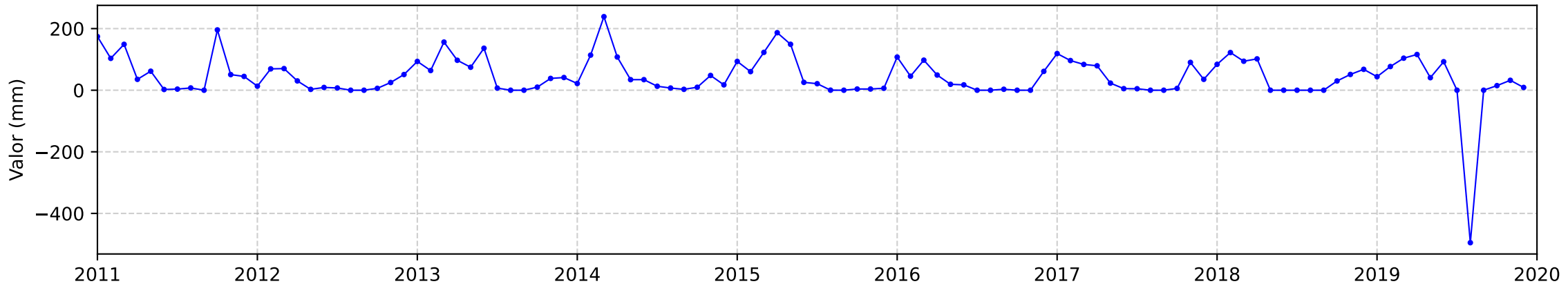
Estação: Barbalha, Década: 2011-2019, Índice: RX5DAY
