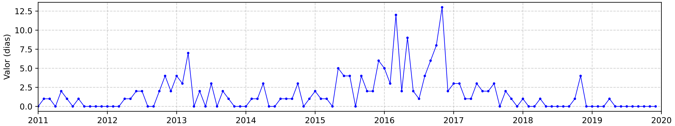
Estação: Barbalha, Década: 2011-2019, Índice: TN90p
