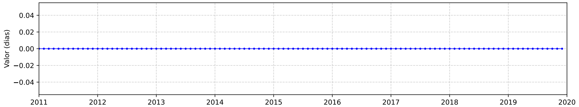
Estação: Barbalha, Década: 2011-2019, Índice: TX10p
