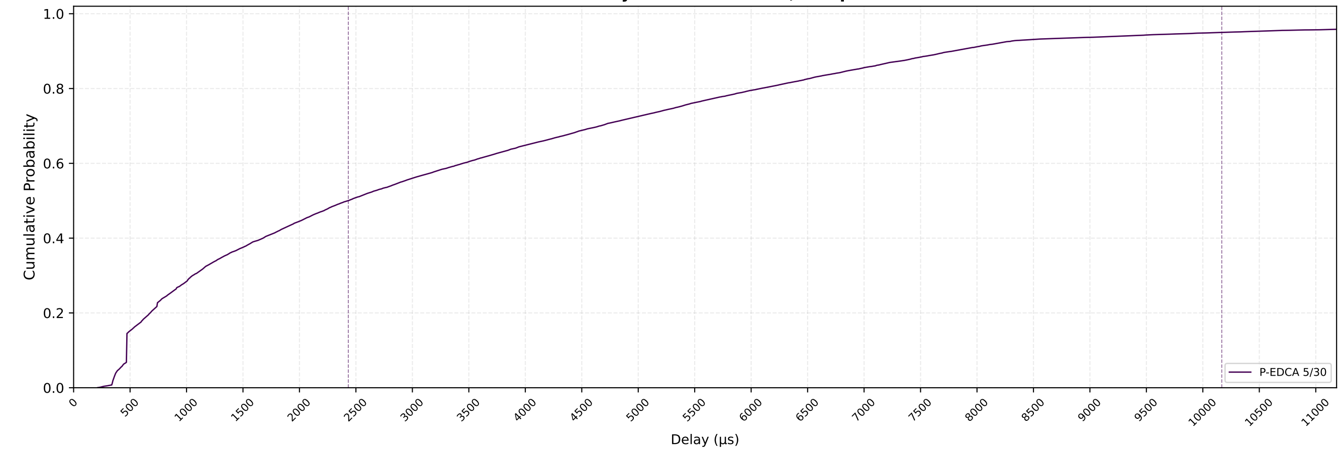
VO Delay CDF — nSta=30, 1Mbps
