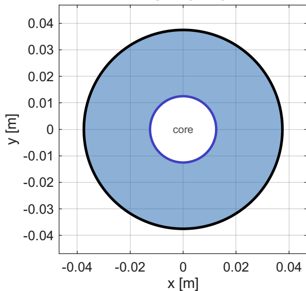
BATES — OD 75mm
