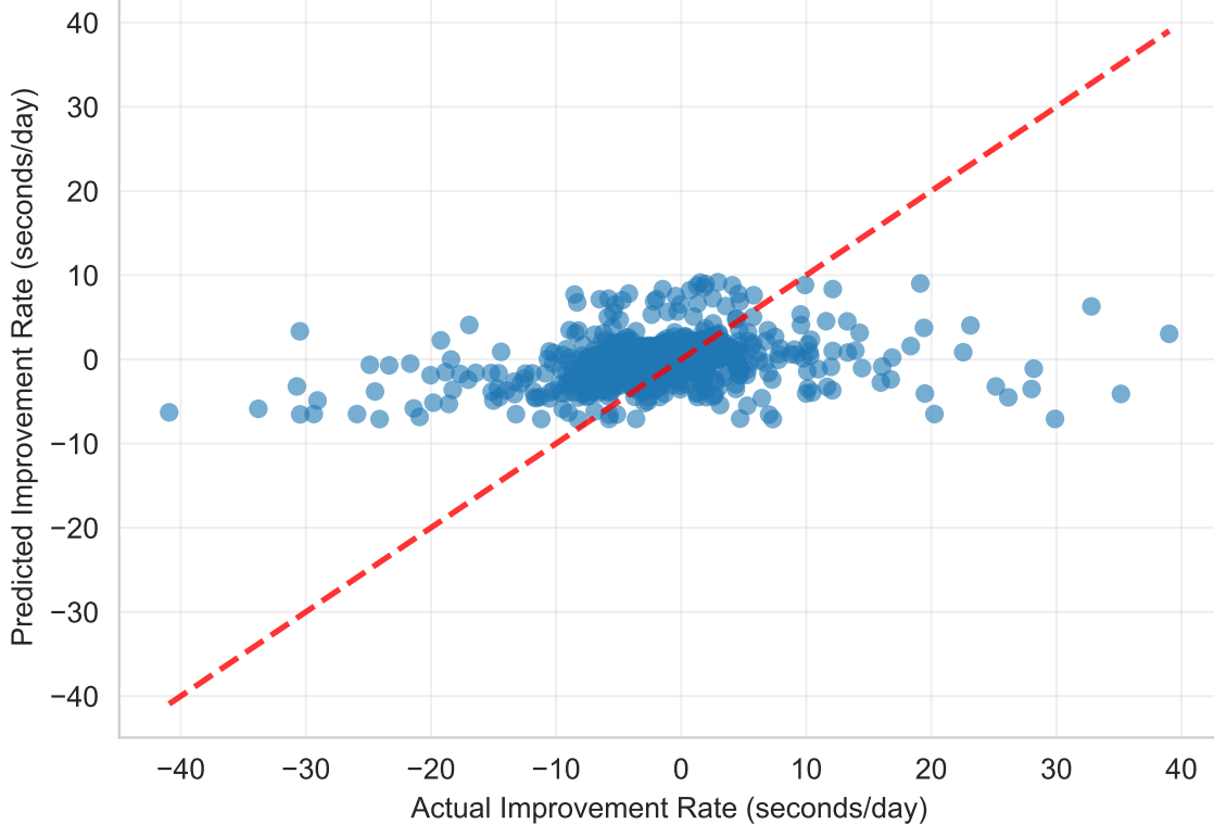
SVR R^2 = 0.038 (95% CI: [-0.030, 0.102]) n=1164
