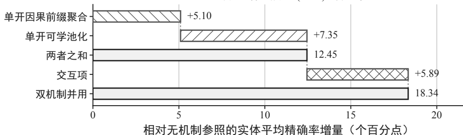
(b) 并用增量按式 (3-30) 的分解
