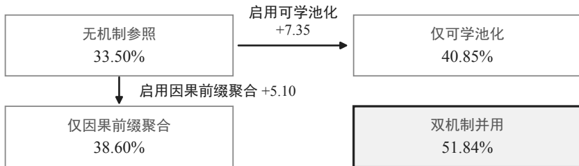
(a) 四格的实体平均精确率与单开一个机制的增量
