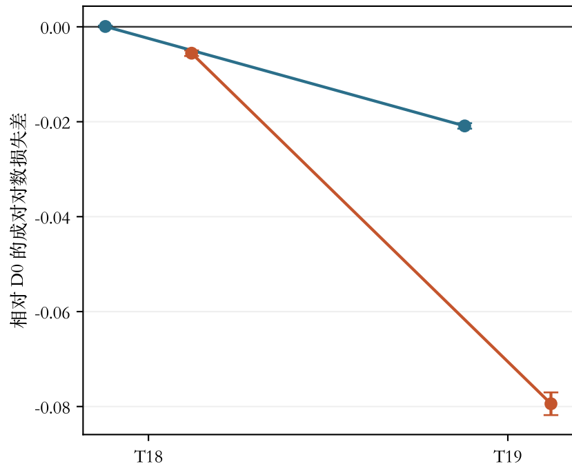
条件记忆键特征的错误预测增量 (95% 区间)
