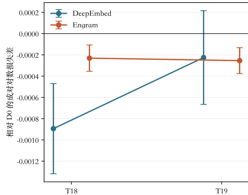
条件记忆键特征的错误预测增量 (95% 区间)
