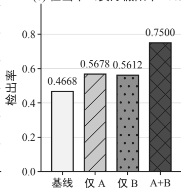
(c) 检出率（实际假阳率 2%）
