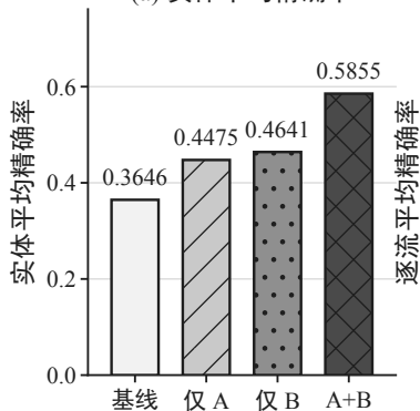
(a) 实体平均精确率
