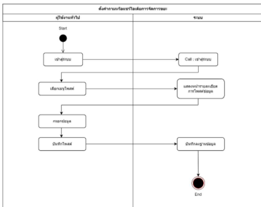
ภาพที่ 32 Activity Diagram ของตั้งคำถามหรือแชร์ไอเดียเดียวการจัดการขยะ
