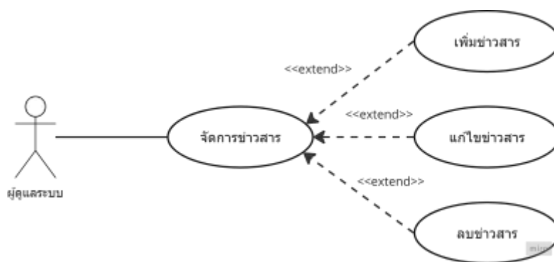
ภาพที่ 23 Use Case Diagram จัดการข่าวสาร
