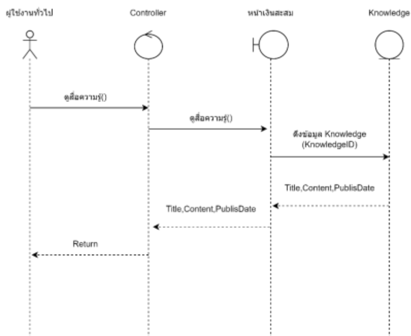
ภาพที่ 48 Sequence Diagram ของดูสื่อความรู้
