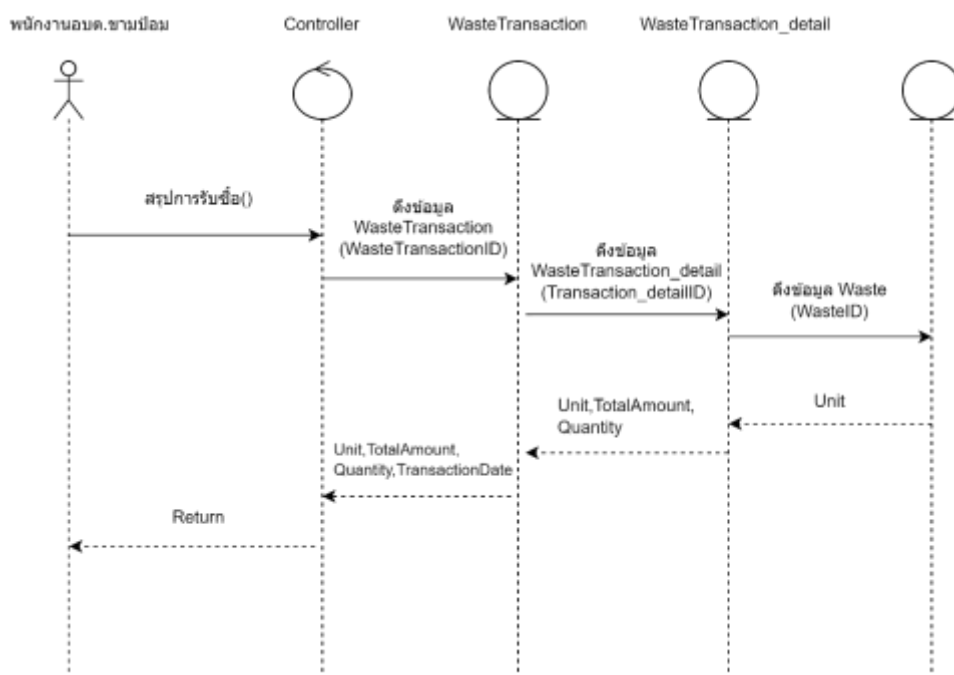
ภาพที่ 53 Sequence Diagram ของเช็คสรุปการรับซื้อ
