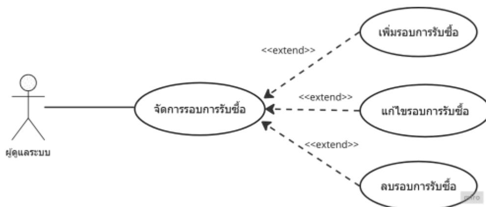
ภาพที่ 27 Use Case Diagram จัดการรอบการรับซื้อ
