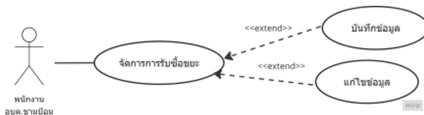
ภาพที่ 14 Use Case Diagram จัดการการรับซื้อขยะ
