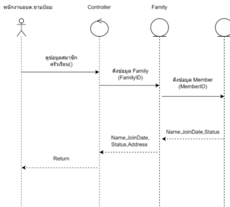
ภาพที่ 54 Sequence Diagram ของจัดการข้อมูลสมาชิกในครัวเรือน
