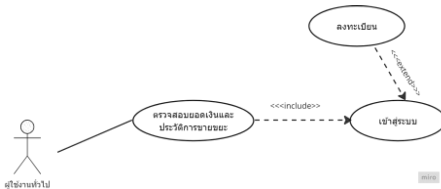
ภาพที่ 9 Use Case Diagram ตรวจสอบยอดเงินและประวัติการขายขยะ
