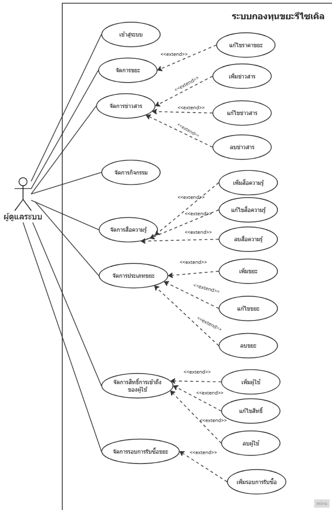
ภาพที่ 8 Use Case Diagram ผู้ดูแลระบบ
