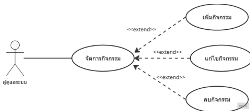
ภาพที่ 25 Use Case Diagram จัดการกิจกรรม
