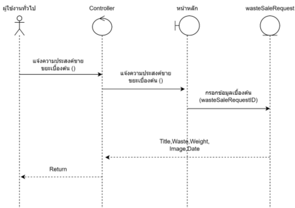
ภาพที่ 50 Sequence Diagram ของแจ้งความประสงค์ขายขยะเบื้องต้น
