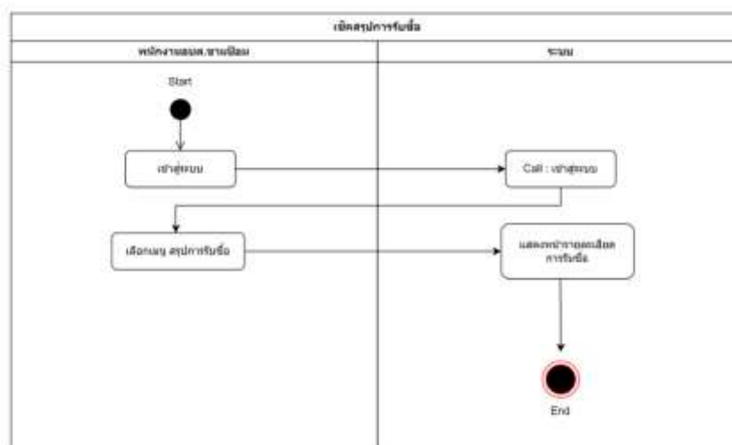
ภาพที่ 36 Activity Diagram ของสรุปการรับซื้อ
