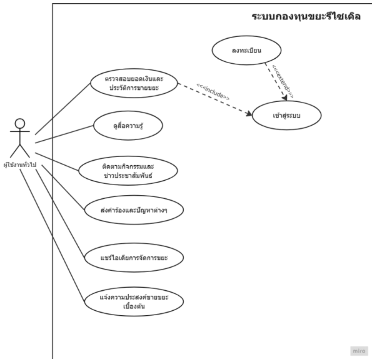
ภาพที่ 6 Use Case Diagram ผู้ใช้งานทั่วไป
