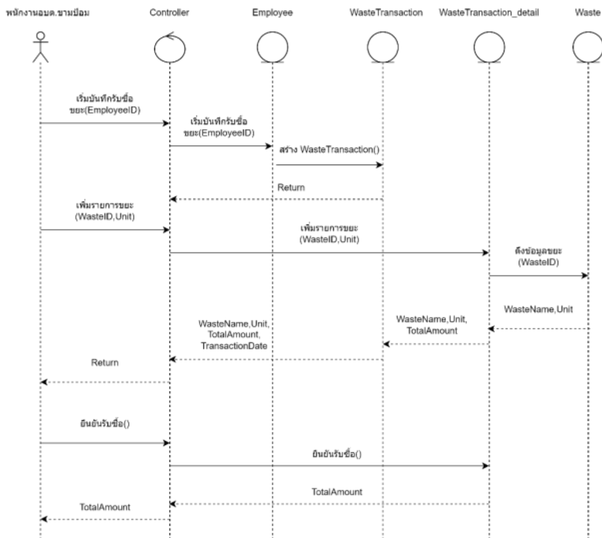
ภาพที่ 51 Sequence Diagram ของจัดการการรับซื้อขยะ
