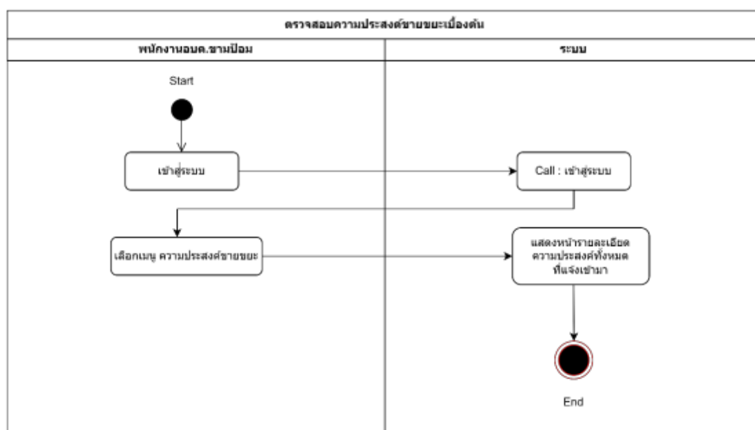
ภาพที่ 41 Activity Diagram ของตรวจสอบความประสงค์ขายขยะเบื้องต้น
