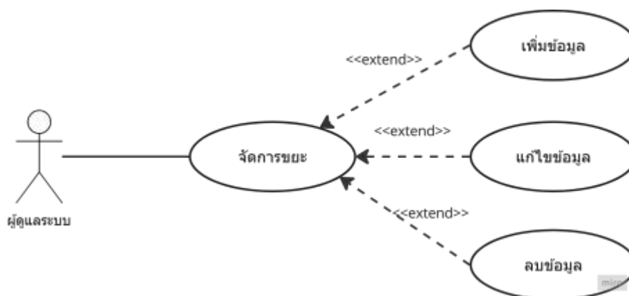
ภาพที่ 22 Use Case Diagram จัดการขยะ
