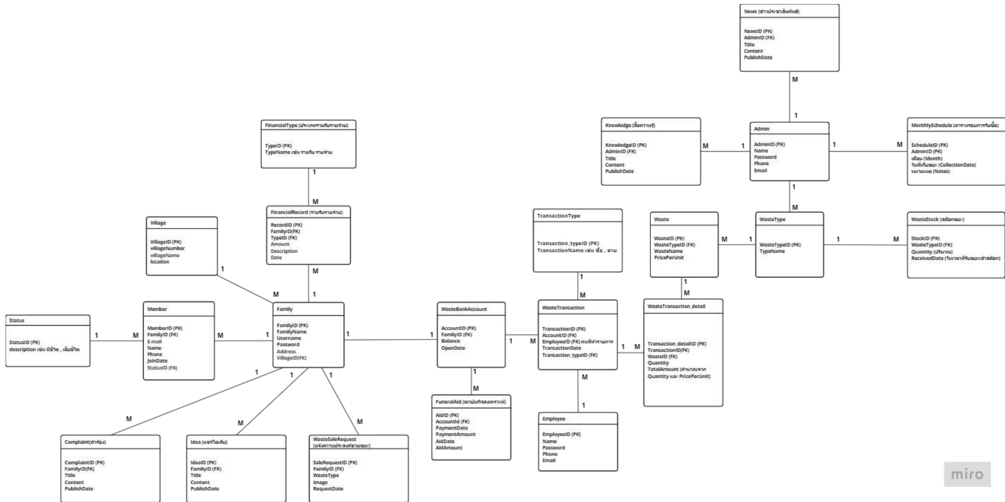
ภาพที่ 63 ER Diagram
