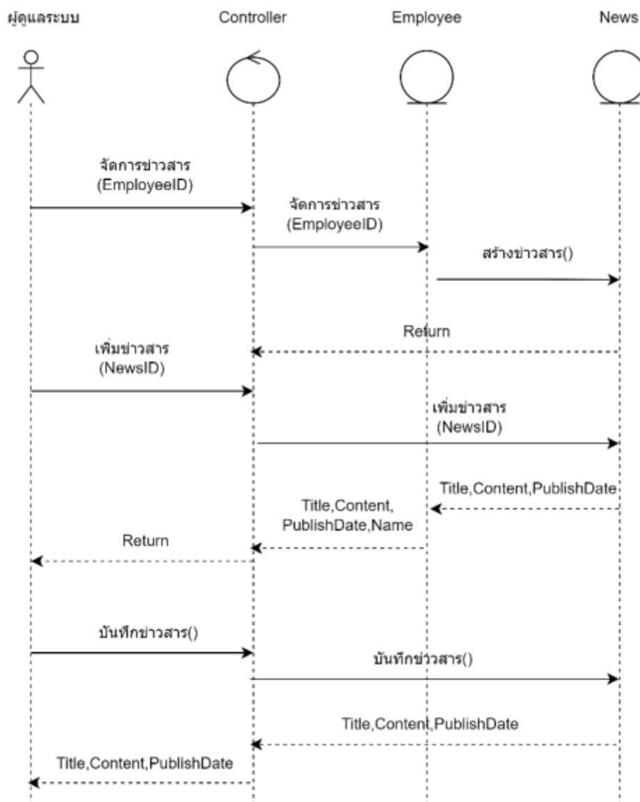
ภาพที่ 59 Sequence Diagram ของจัดการข่าวสาร
