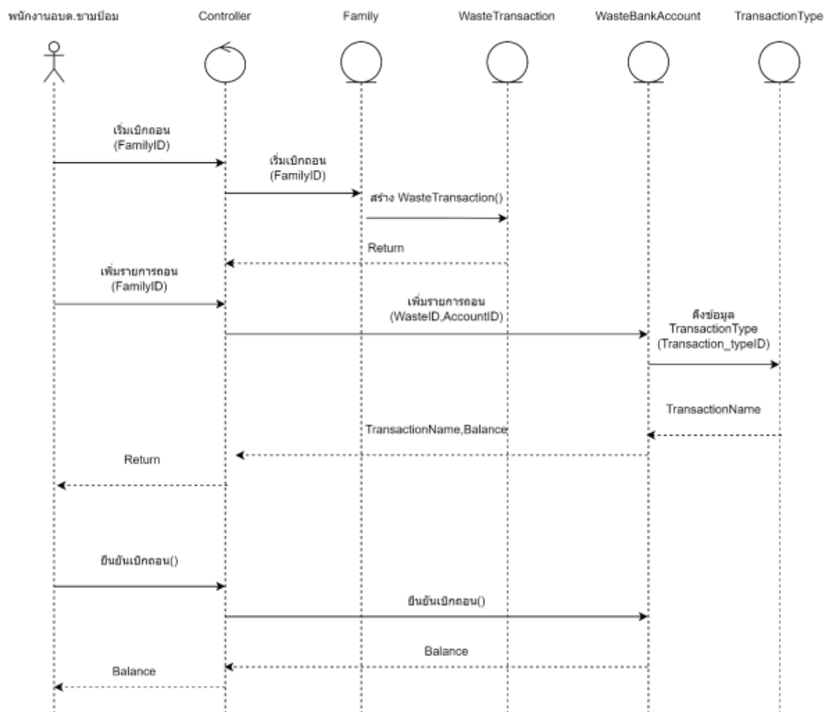
ภาพที่ 56 Sequence Diagram ของจัดการข้อมูลการเบิกถอน
