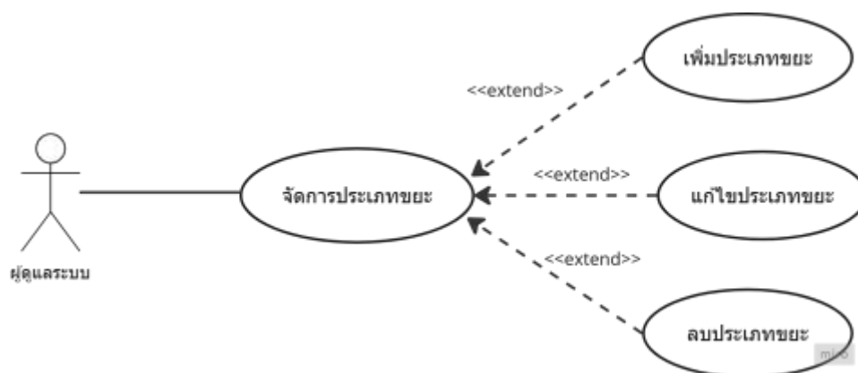
ภาพที่ 26 Use Case Diagram จัดการประเภทขยะ
