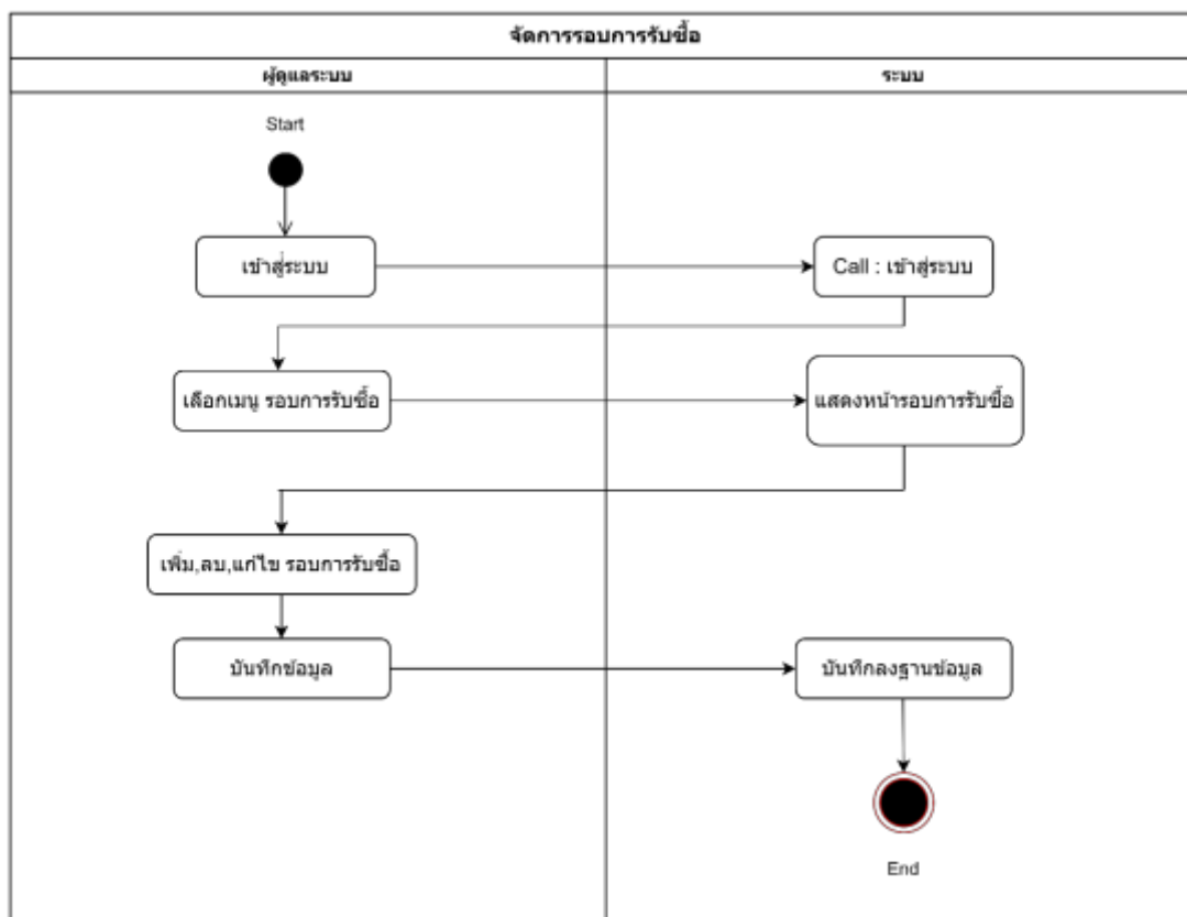
ภาพที่ 46 Activity Diagram ของจัดการรอบการรับซื้อ
