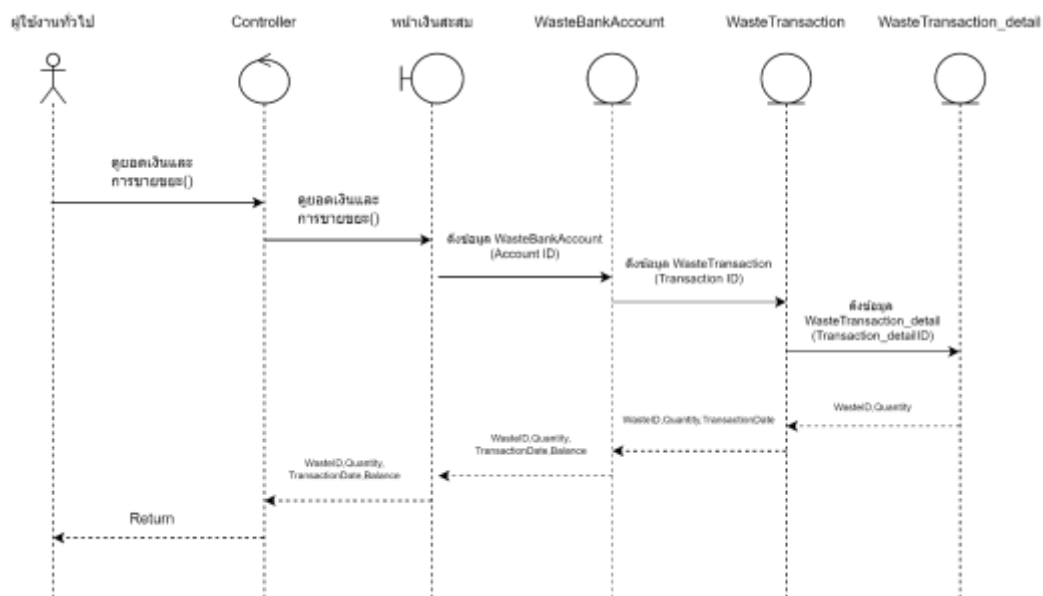
ภาพที่ 47 Sequence Diagram ของตรวจสอบยอดเงินและประวัติการขาย
