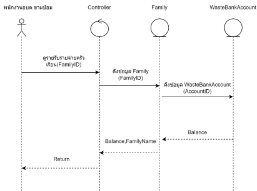
ภาพที่ 55 Sequence Diagram ของจัดการข้อมูลรายรับรายจ่ายของครัวเรือน
