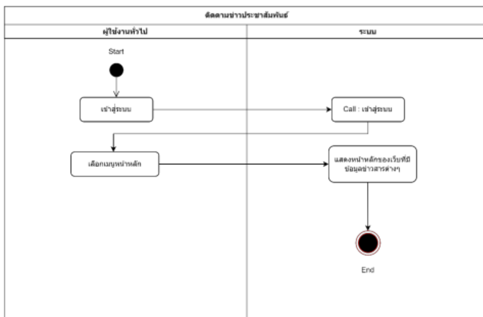
ภาพที่ 30 Activity Diagram ของติดตามความประชาสัมพันธ์
