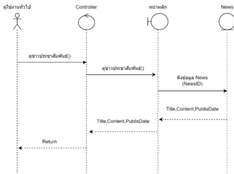
ภาพที่ 49 Sequence Diagram ของติดตามข่าวประชาสัมพันธ์
