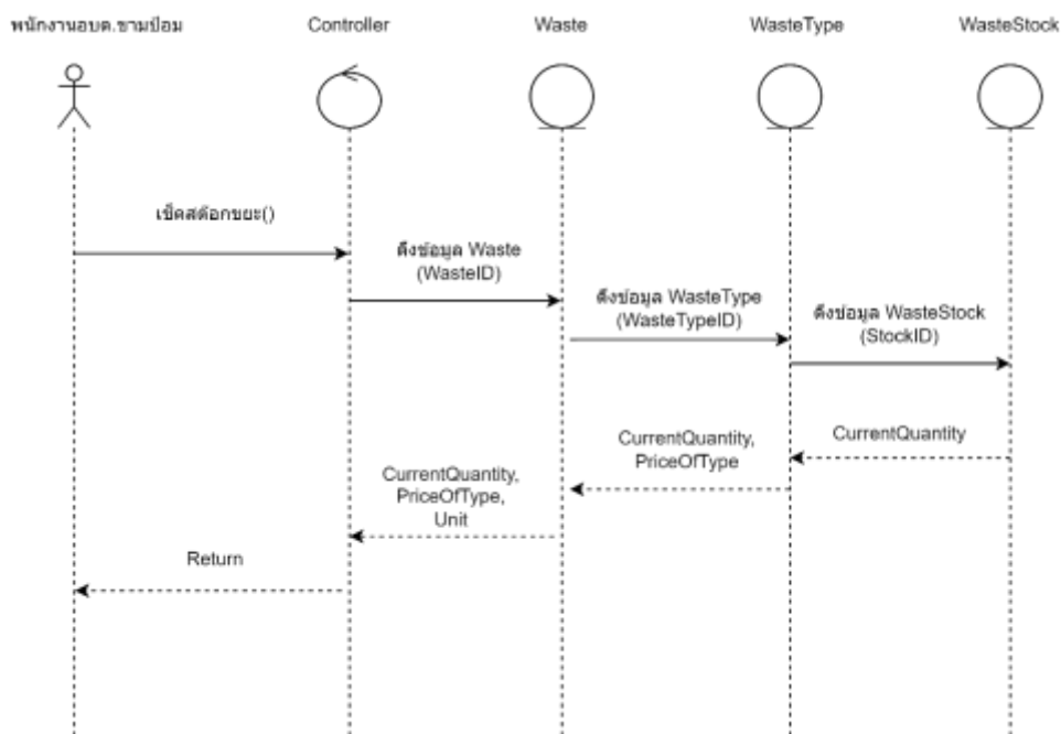
ภาพที่ 52 Sequence Diagram ของเช็คสต็อกขยะ
