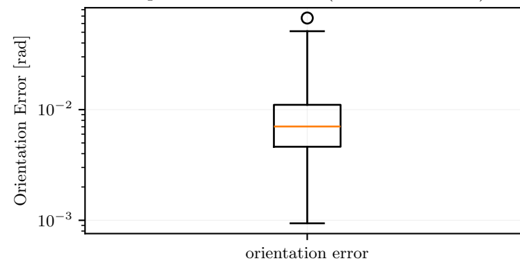
Tip Orientation Error (PINN - Cosserat)
