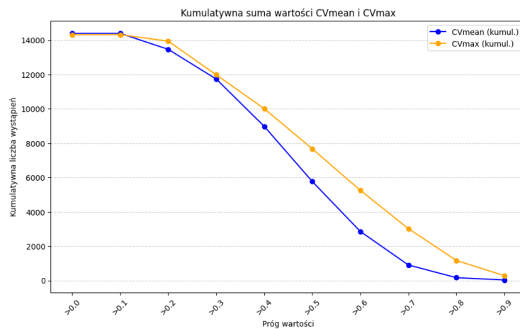
Rysunek 4: Kummulatywny wykres CV
