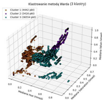
Rysunek 15: Wizualizacja klastrowania Warda na 3 klastry – brak wyraźnego podziału między różnymi typami nieba.
