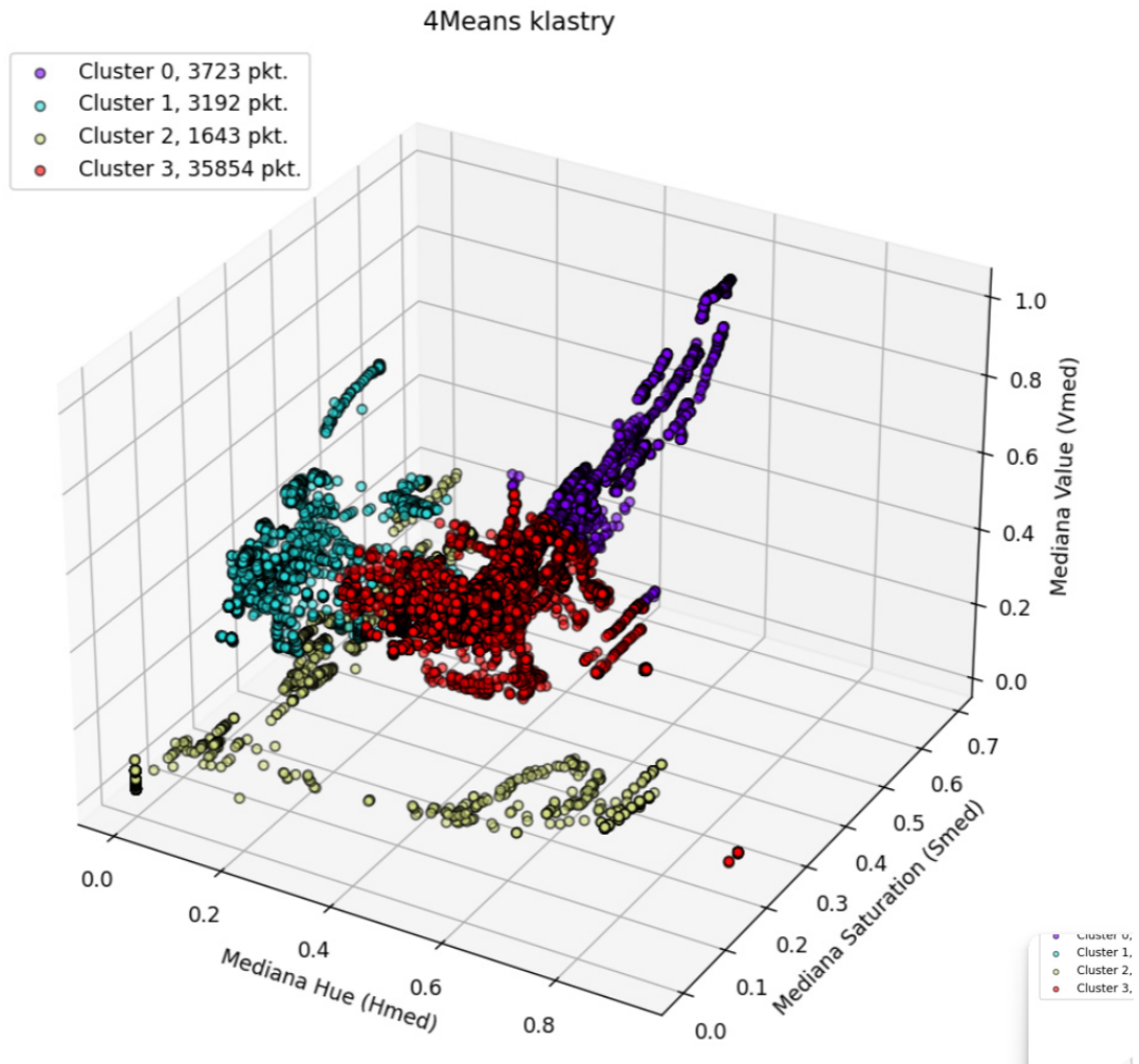
Rysunek 8: Wyniki KMeans dla wektora \vec{f}_2 : wizualizacja 3D klastrów i ich etykiet interpretacyjnych.
