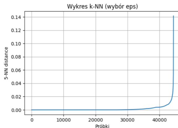
Rysunek 10: Wykres 5-NN dla danych z wektorem \vec{f}_2 – wybór parametru \text{eps} .
