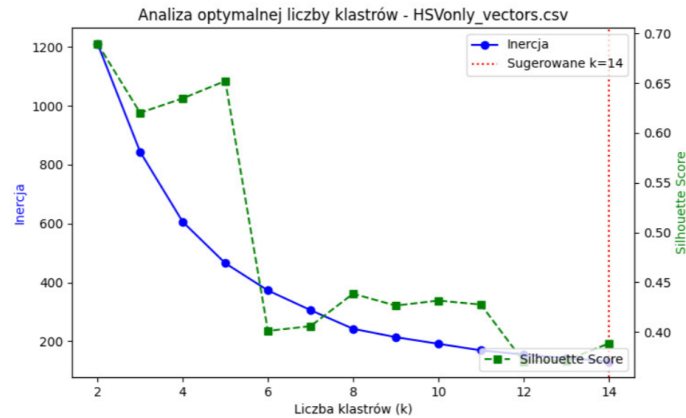
Rysunek 7: Analiza optymalnej liczby klastrów na podstawie inercji i wskaźnika silhouette dla wektora \vec{f}_2 .
