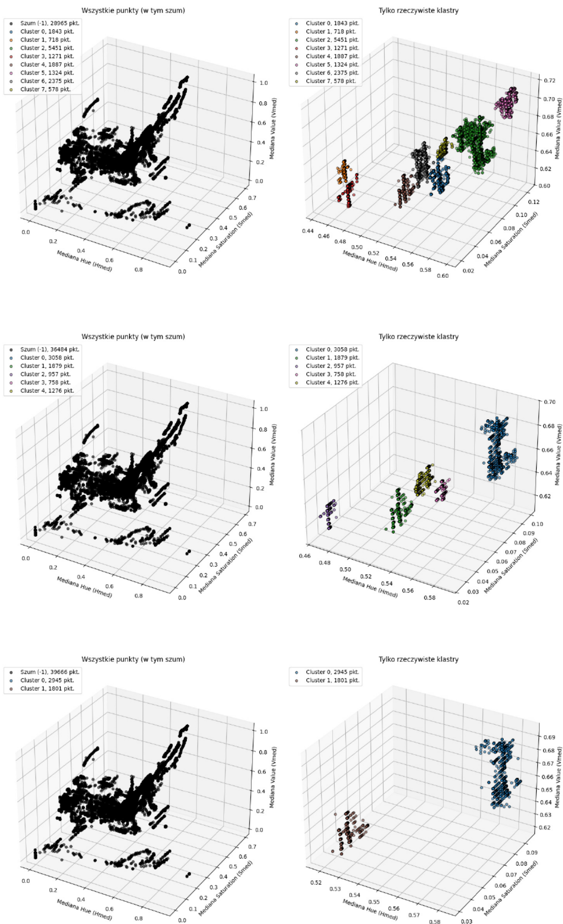
Rysunek 10: Więcej wyników klastrowania DBSCAN dla \vec{f}_2^- .
