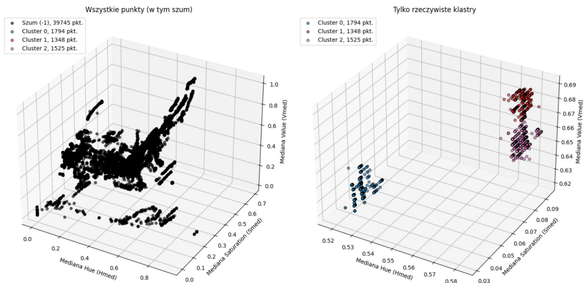
Rysunek 9: Wyniki klastrowania DBSCAN dla \vec{f}_2 – u góry: zidentyfikowane 3 klastry, u dołu: 2 klastry. Po lewej – wszystkie punkty, po prawej – tylko klastry (bez szumu).
