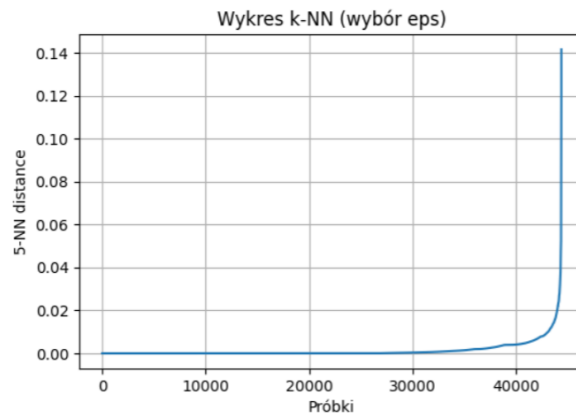
Rysunek 8: Wykres 5-NN dla danych z wektorem \vec{f}_2 – wybór parametru \text{eps} .
